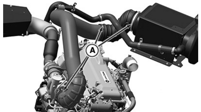
Moteur de turbocompresseur à simple étage
