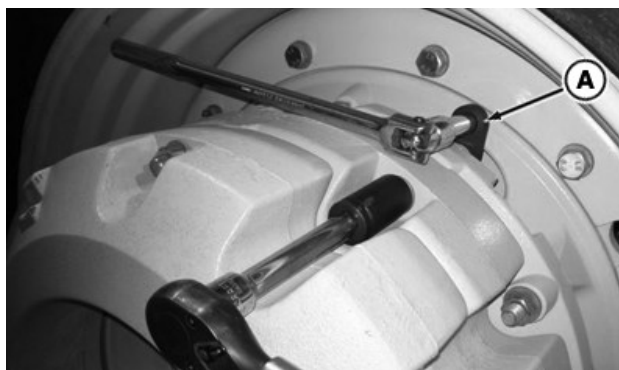
Masse de lestage de roue extérieure
