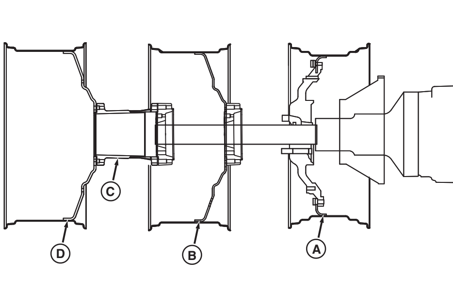
Moyeux de roue renforcés
