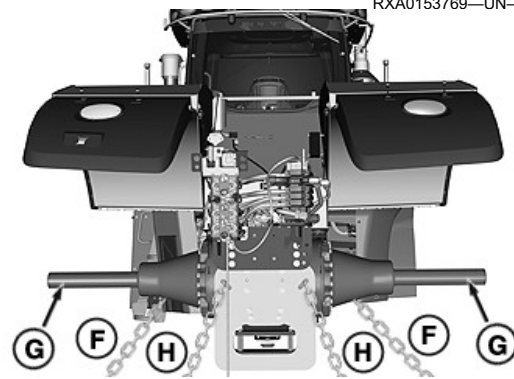
Attelage du racleur
