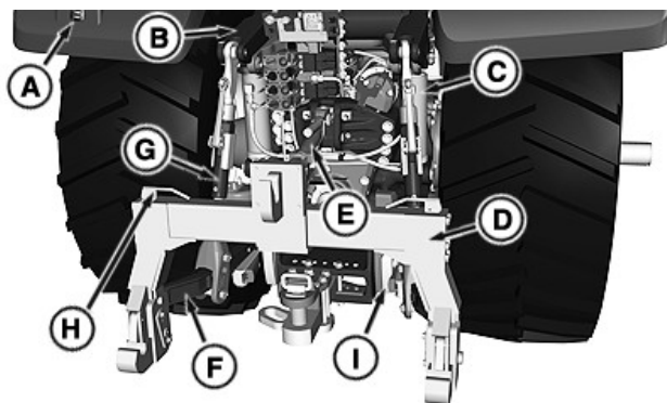
Composants de l'attelage arrière
