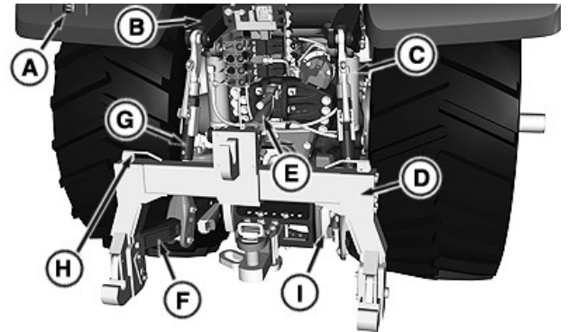
Composants de l'attelage arrière
