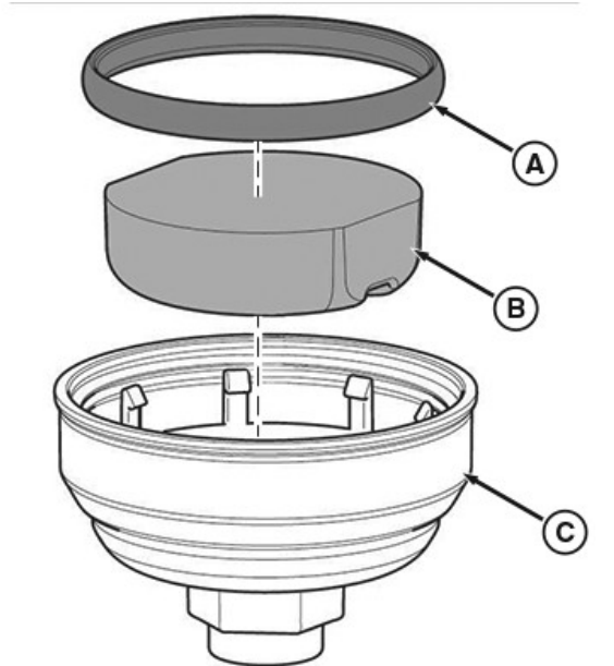
Componentes de la caja del filtro
