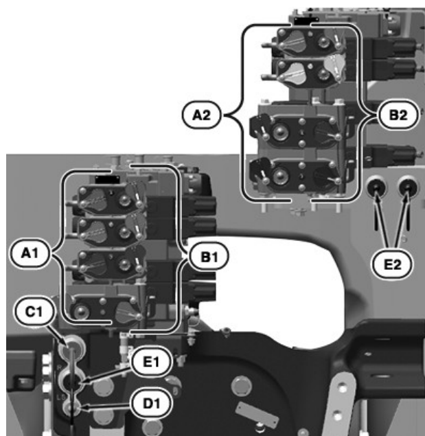
RXA0178746—UN—17NOV20 Bloque de VMD del sistema hidráulico de caudal alto— Ocho VMD con toma exterior hidráulica en la fundición del enganche
