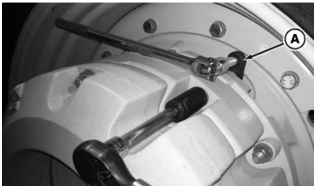
Contrapesos exteriores de ruedas
