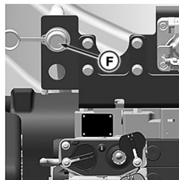
RXA0187065—UN—13APR22 Identificación y ubicación de los componentes [Ag]— Sistema hidráulico de caudal alto: (F) Acoplador del sumidero—Vaciado del cárter del motor
