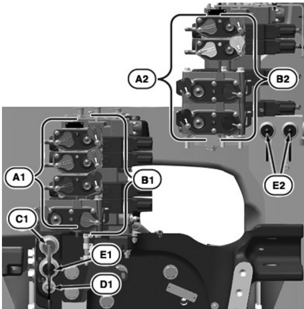
Bloque de VMD del sistema hidráulico de caudal alto— Ocho VMD con toma exterior hidráulica en fundición de enganche
