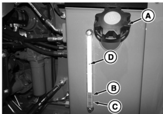
Mirilla de aceite hidráulico
