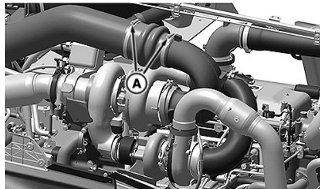
RXA0180399—UN—10NOV20 Sistema de admisión de aire—Lado derecho
