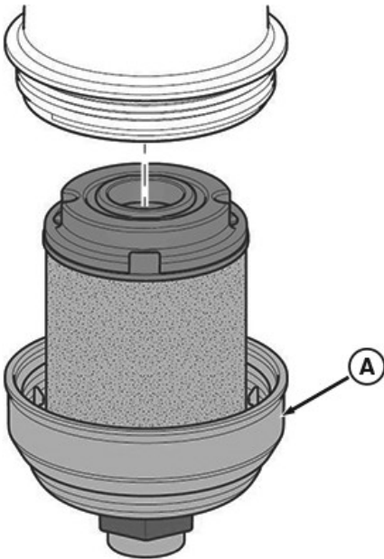
RG30727—UN—08AUG18 Extracción del filtro
