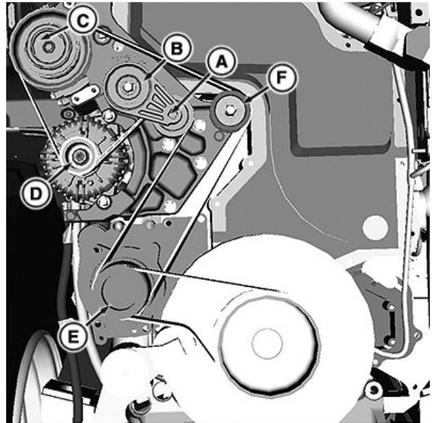
Disposición de la correa de transmisión auxiliar
