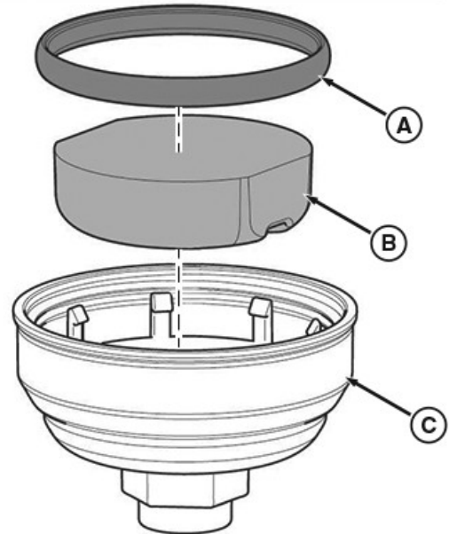
RG30726—UN—08AUG18 Componentes de la caja del filtro
