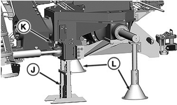
Tope de oscilación y soportes de apoyo
