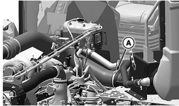
RXA0180449—UN—19NOV20 Sistema de admisión de aire—Lado izquierdo
