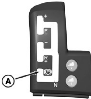
RXA0140499—UN—16APR14 Posición de ESTACIONAMIENTO de la palanca del inversor con mando en lado derecho
