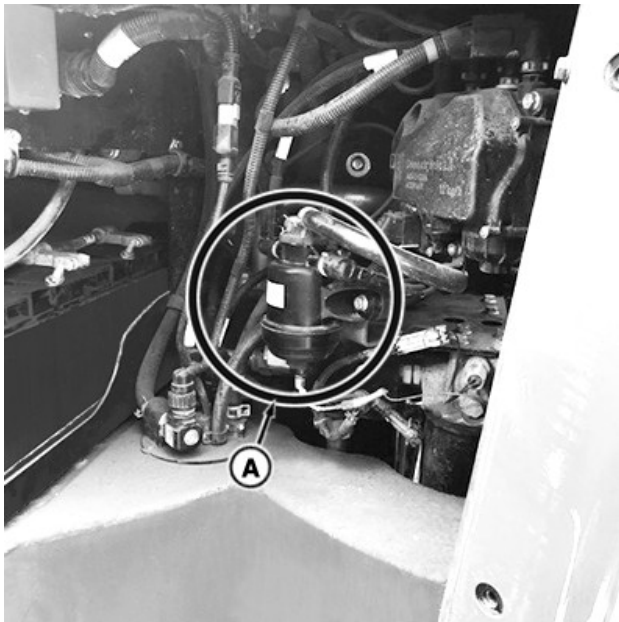
RXA0163952—UN—24JUL18 El filtro en línea de fluido de escape diésel (DEF) (A) está dentro del compartimento de la batería.
