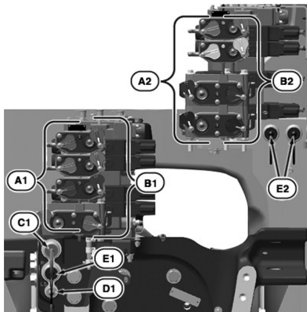
RXA0178746—UN—17NOV20 Bloque de VMD hidráulico de caudal alto
