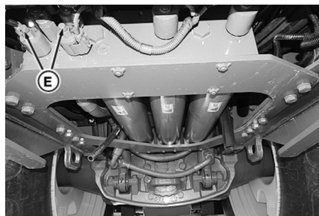
Hydraulické elektromagnetické ventily (umístěné pod předním rámem)
