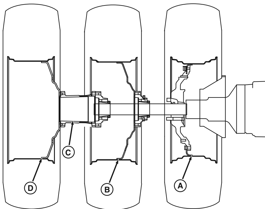
Trojítá kola (standardní náboje kol)
