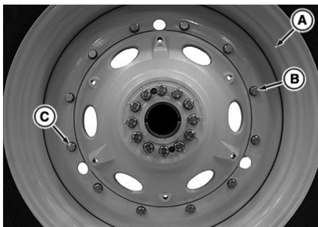
Kolo s 12 šrouby s pouzdry nábojů s dvojitým úkosem
