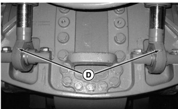
Dolní maznice odpruženého zavěšení nápravy
