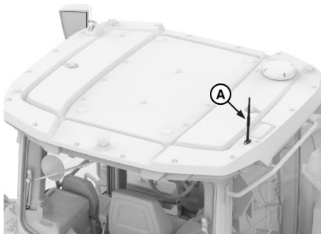
Umístění antény pro synchronizaci strojů John Deere
