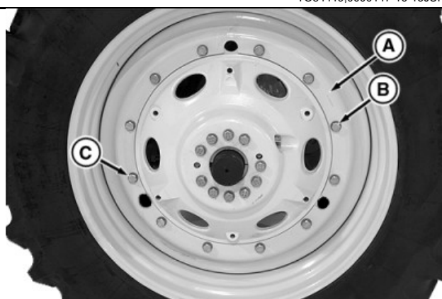
Kolo s 10 šrouby
