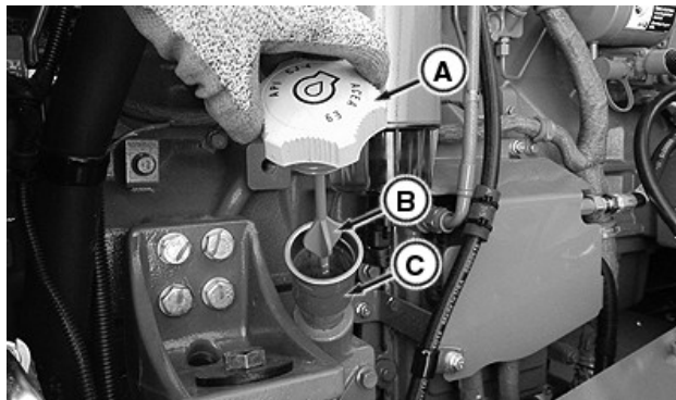
Motor 13,5 l
