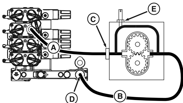
Striekacie čerpadlo (bez závesu)
