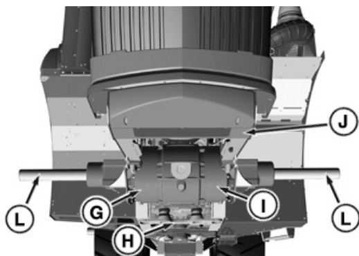
Zdvíhacie body (na prednej strane)
