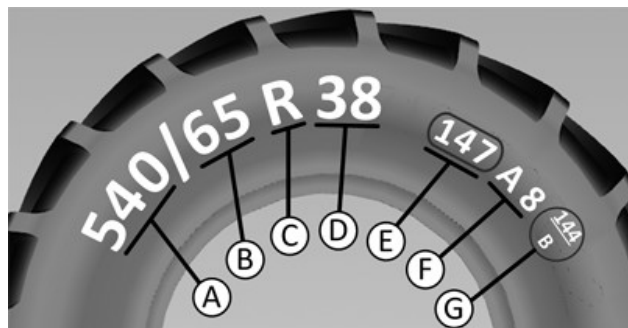
Príklad informácií výrobcu na bočnej strane pneumatiky
