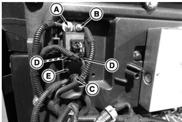
Modul relé napájania náradia
