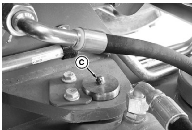
Ľavý predný čap riadenia
