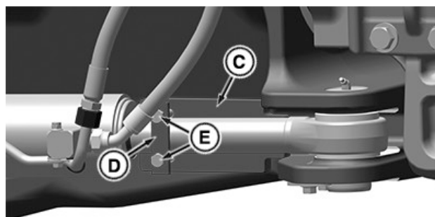
Namontovaný zámok riadenia (ľavá strana)
