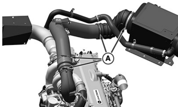
RXA0188967—UN—17MAY23 Dvojstupňový turbo motor
