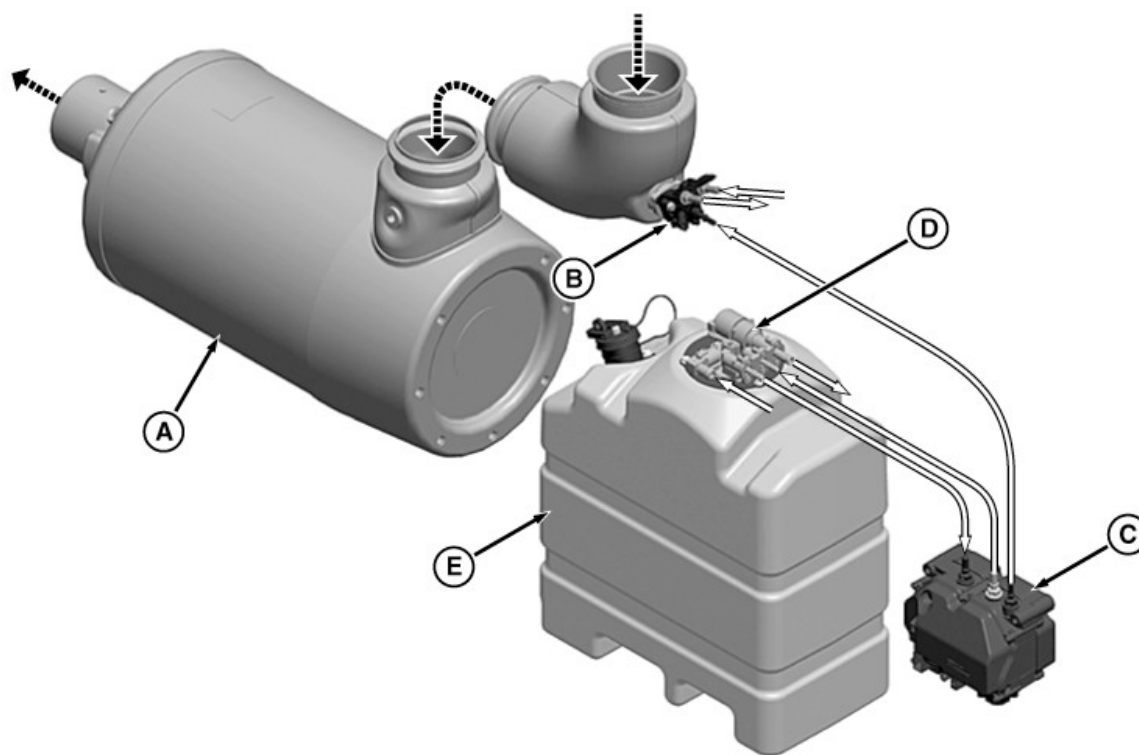
Sústava SCR
