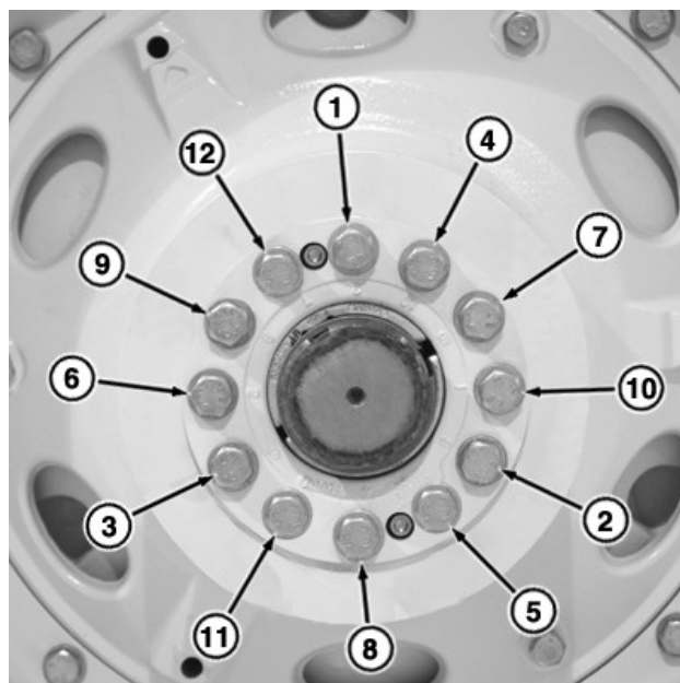
RXA0090157—UN—08AUG06 Postup uťahovania: Zostava náboja hnacieho kolesa pre vysokú záťaž s dvomi kuželmi
