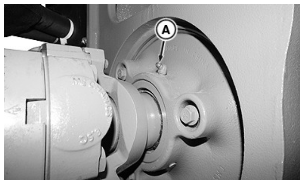
Prípojka ložiska hnacieho ústrojenstva otočného čapu
