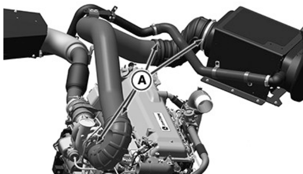
RXA0188966—UN—17MAY23 Jednostupňový turbo motor
