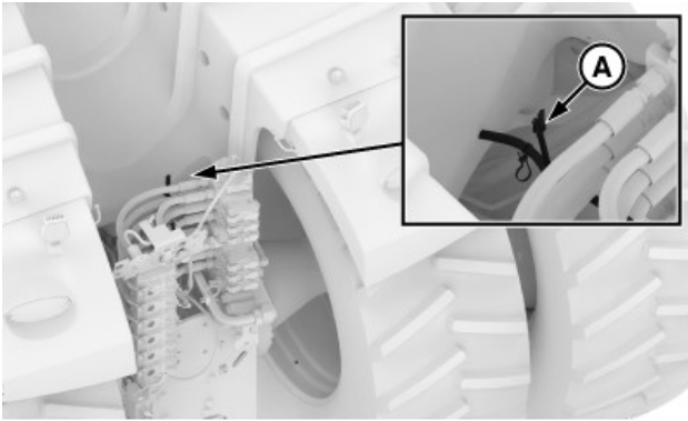
Prípojka kabeláže snímača zaťaženia
