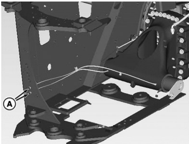
Axelfjädring, diagram över bakre bussningar
