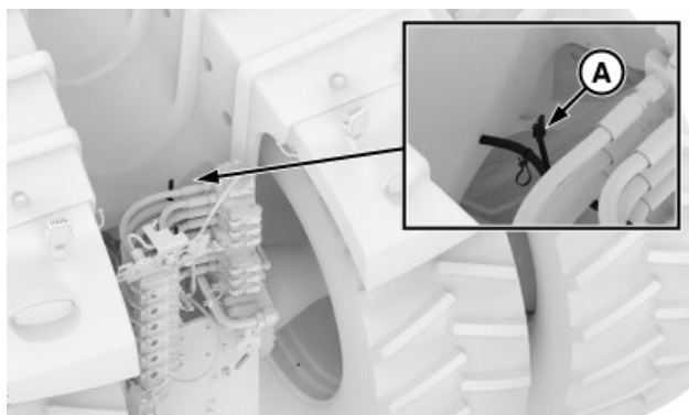
Dragkraftsgivarens kabelanslutning
