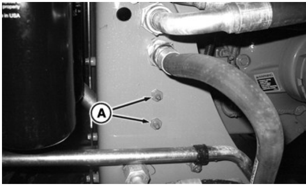
Bussningar bak, HydraCushion™-framaxel
