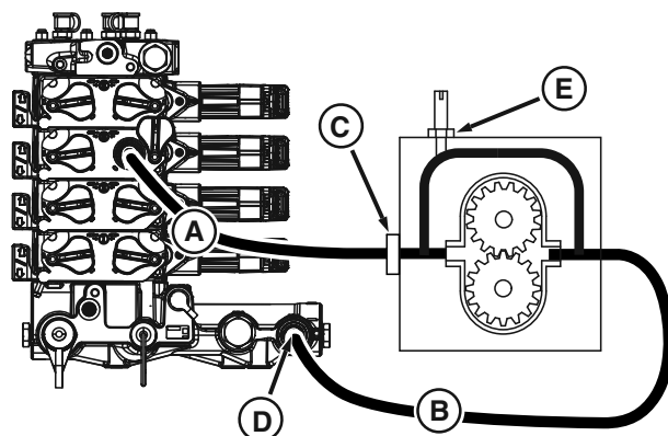
Sprutpump—Utan lyft
