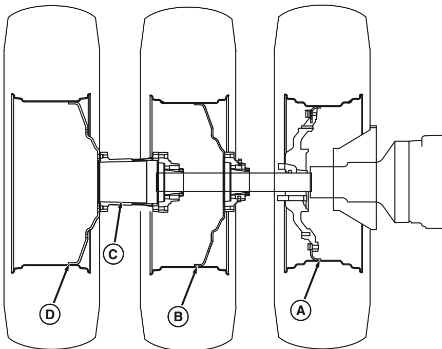
Tredubbla hjul (standardhjulnav)
