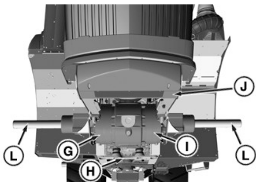
RXA0188398—UN—20DEC22 Lyftpunkter (framtill)
