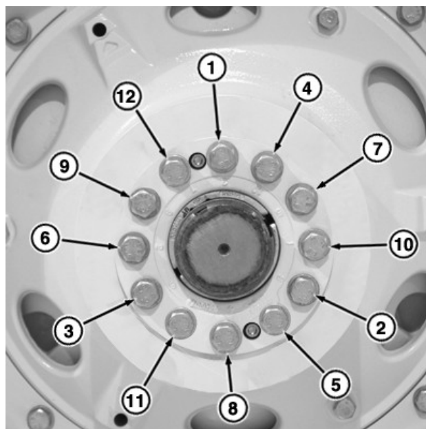
RXA0090157—UN—08AUG06 Åtdragningsföljd: Dubbelt koniska kraftiga drivhjulsnäv
