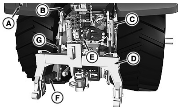
Lyftkomponenter
