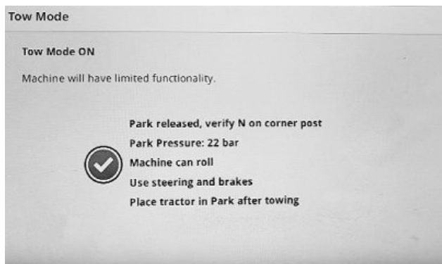
Parkeringsstryck i bogseringsfunktion
