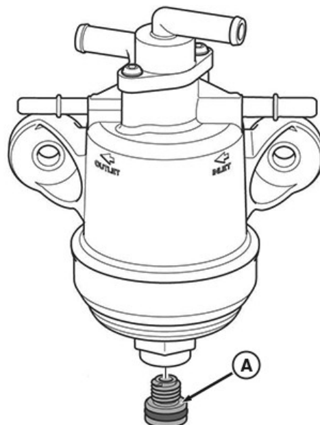
RG30728—UN—08AUG18 Korek spustowy filtra liniowego DEF
