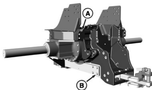
Wspornik wzmacnionego zaczepu rolniczego - oś z pojedynczą redukcją
