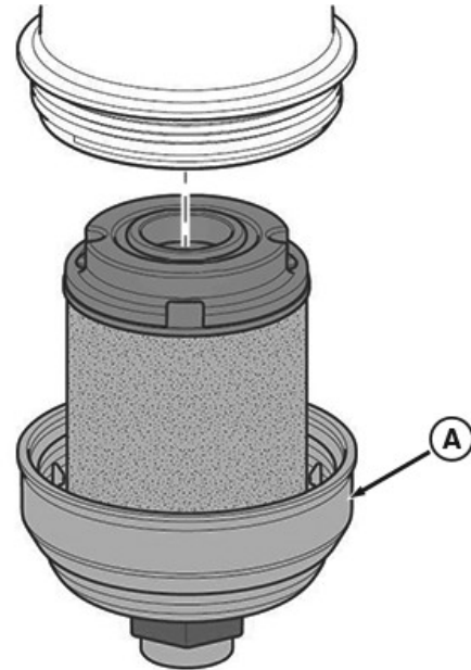
RG30727—UN—08AUG18 Montaż obudowy filtra liniowego DEF
