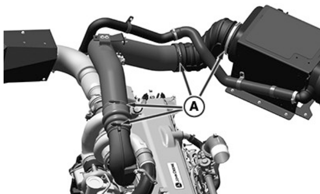
Silnik z podwójną turbosprężarką RXA0188967—UN—17MAY23
