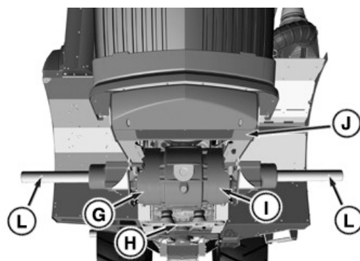
Punkty podnoszenia (z przodu)
