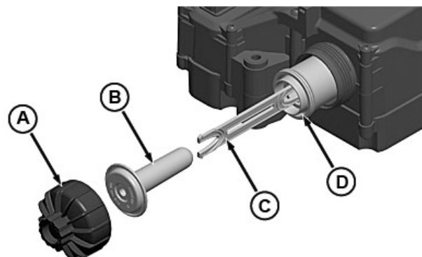
Filtr modułu dawkowania DEF
