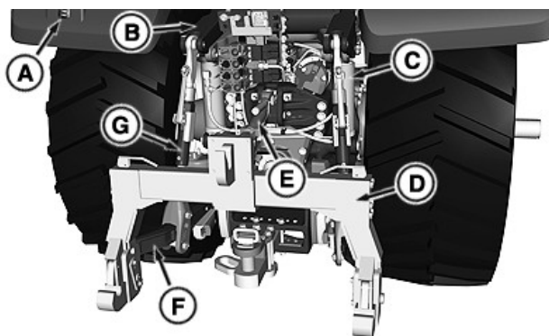
Podzespoły podnośnika
