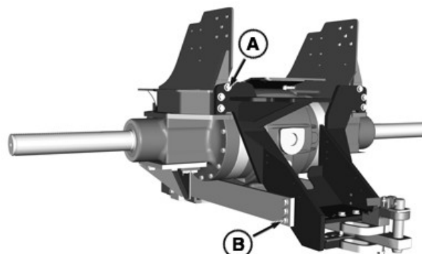
Wspornik standardowego zaczepu rolniczego - oś z pojedynczą redukcją
