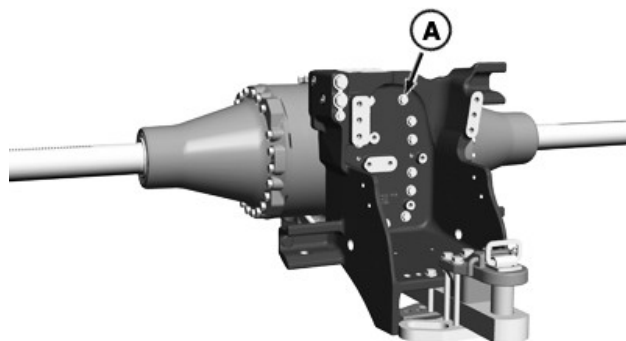
Wspornik wzmacnionego zaczepu rolniczego - oś z podwójną redukcją
