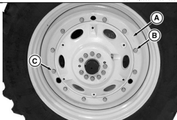
Koło z 10 śrubami
