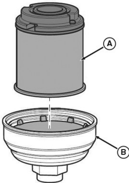
RG30725—UN—08AUG18 Montaż obudowy i elementów filtra
