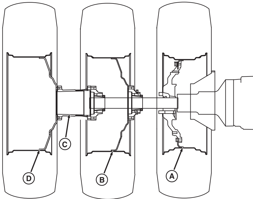
Koła potrójne (standardowe piasty kół)
