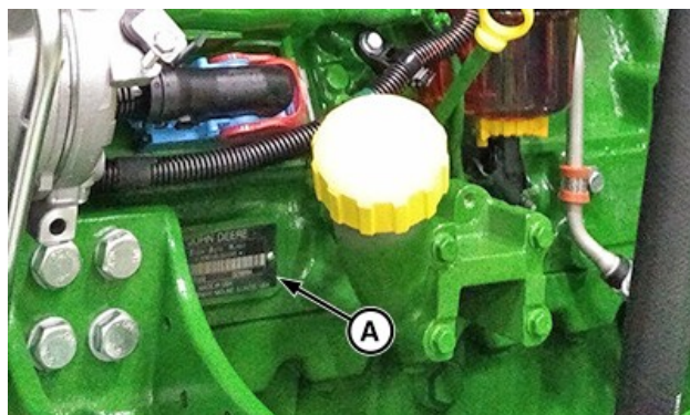
Tabliczka z numerem seryjnym silnika (A) (części zdemontowane do celów ilustracyjnych)
