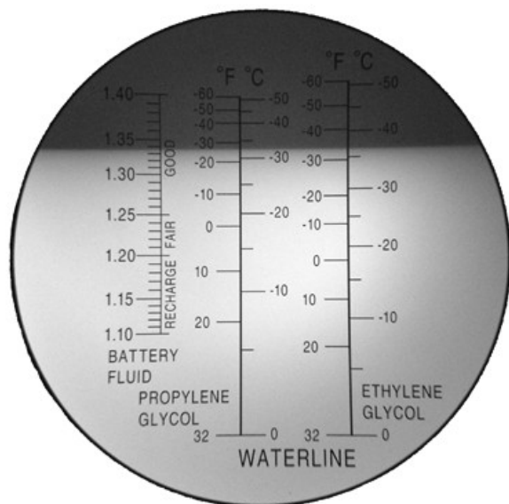
TS1733—UN—04SEP13 Imagine cu o picătură de lichid de răcire 50/50 pe fereastra refractometrului
