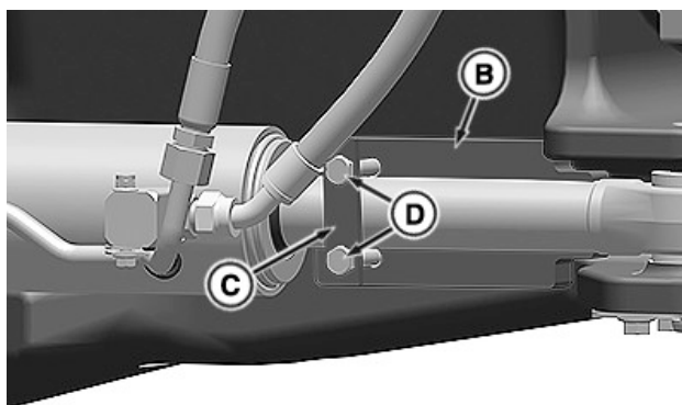
RXA0188672—UN—23FEB23 Dispozitiv de blocare a direcției instalat (partea stângă)
