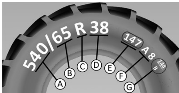
Exemplu de informații oferite de producători pe peretele lateral
