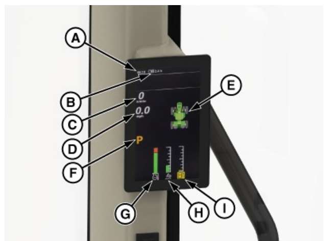
RX1361839—UN—27MAR24 Afișajul de pe consola din colț
