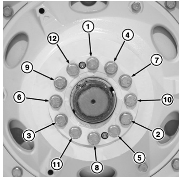
RXA0090157—UN—08AUG06 Ordinea de strângere: Ansamblul butucului de regim greu cu conic dublu roată motoare
