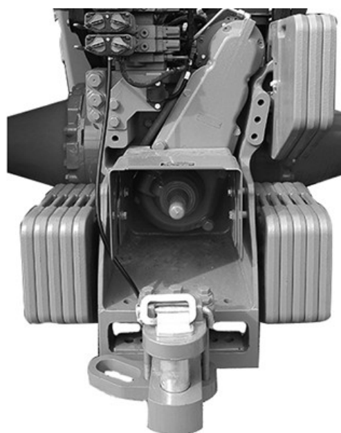
Configurarea lestării maxime cu priză de putere
