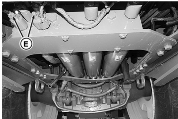
RXA0160220—UN—17JUL17 Electrovalvele hidraulice (amplasate sub cadrul din față)
