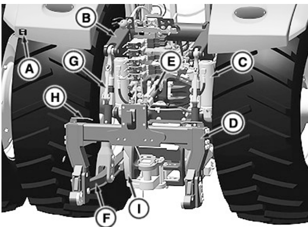
Componentele cârligului din spate
