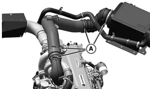
Motor cu turbosuflantă cu două trepte
