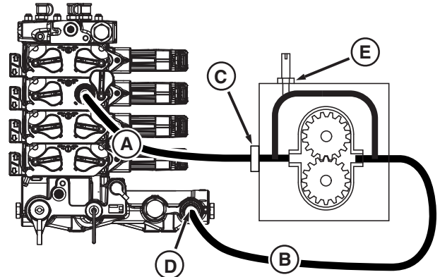
Pompă de stropire—fără cuplaj
