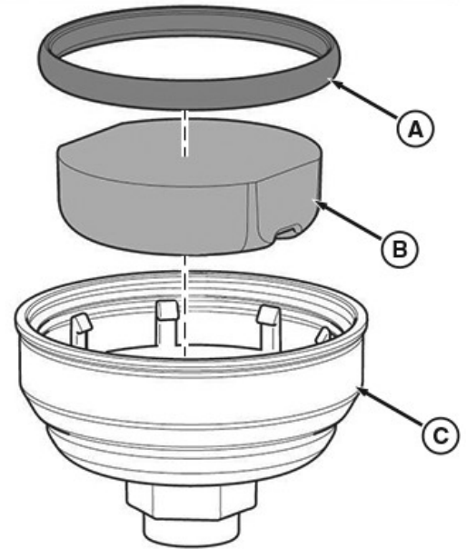
RG30726—UN—08AUG18 Componentele carcasei filtrului
