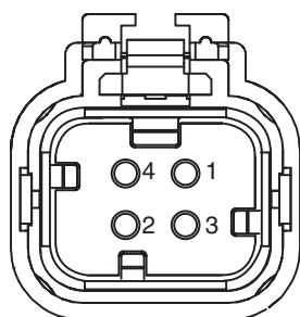
Identificazione dei contatti del connettore video
