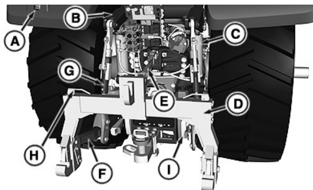
Componenti del sollevatore posteriore
