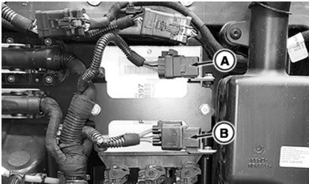
RXA0180458—UN—17NOV20 I relè del modulo relè di alimentazione dell'attrezzatura sono nell'angolo superiore destro del pannello posteriore della cabina.
