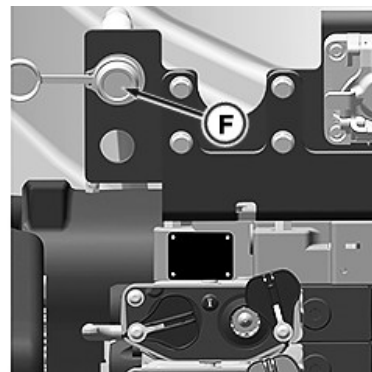
Identificazione dei componenti e ubicazione [Ag]—Sistema idraulico ad alta portata: (F) Attacco della coppa—Scarico della scatola del motore
