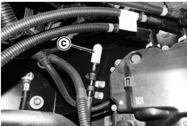
Il filtro di sfiato del serbatoio DEF (C) si trova nel vano batteria sopra l'unità di dosaggio DEF.
