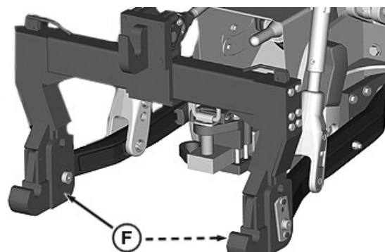
Sollevatore rapido mostrato nella configurazione di categoria 4N
