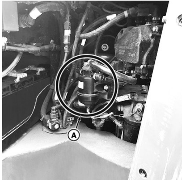
Il filtro in linea DEF (A) si trova all'interno del vano batteria.
