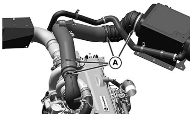
Motor cu turbosufletă cu două trepte
