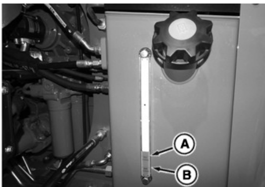
Vizor pentru rezervorul de ulei hidraulic
