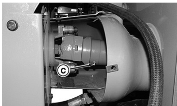
Fitingul arborelui prizei de putere spate (cu piese demontate)
