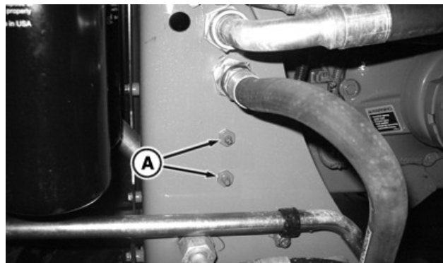
Bucșe spate punte față HydraCushion™
