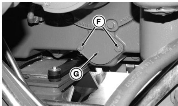
Pāresumkārbā, skats no aizmugures
