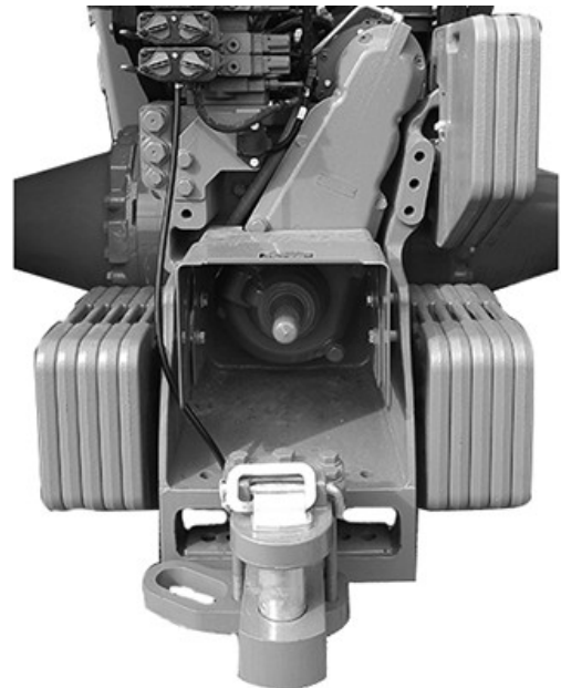
Maksimālā balasta konfigurēšana ar jūgvārpstu
