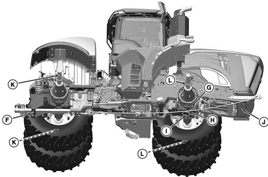
Pacelšanas punkti (apakšpuse ar [Ag] jūgstieni)
