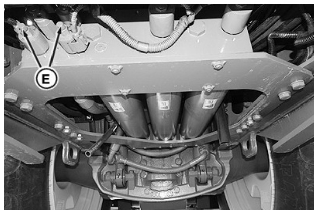
RXA0160220—UN—17JUL17 Hidraulikas solenoīdu vārsti (atrodas zem priekšējā rāmja)
