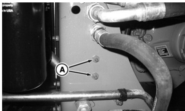
Priekšējās ass “HydraCushion”™ aizmugurējās bukses
