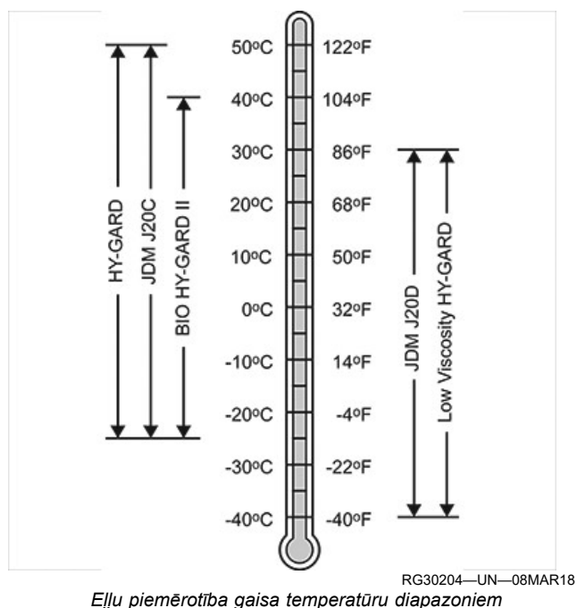
Eļļu piemērotība gaisa temperatūru diapazoniem
