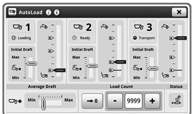
AutoLoad piemērs
