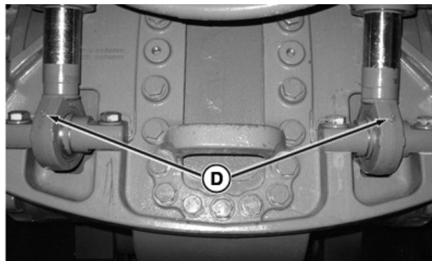
Ass apakšējās daļas balstiekārtas nipeļi
