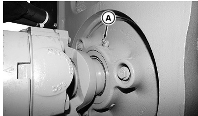
Spēka pārvada šarnīra gultņa smērnipeļis
