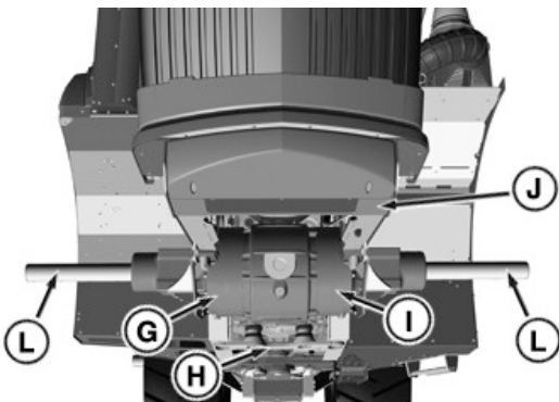
RXA0188398—UN—20DEC22 Celšanas punkti (priekšā)
