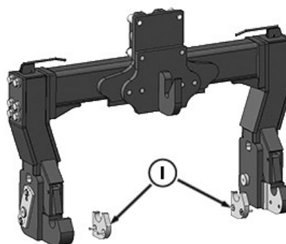
RXA0184176—UN—22JUN21 Parādīta ātrā sakabe ar 3. kategorijas āķi
