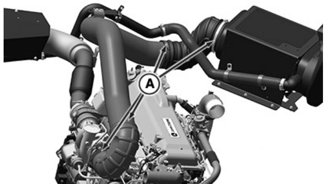
Vienas pakāpes turbo dzinējs
