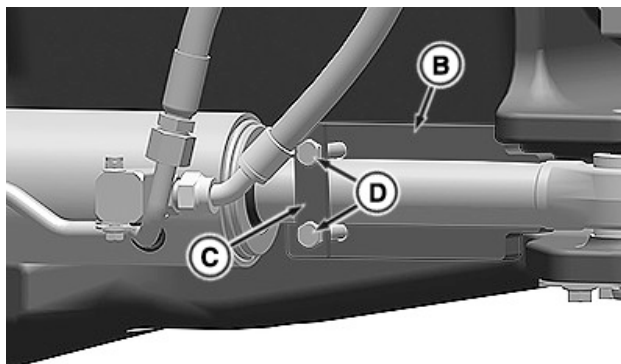
RXA0188672—UN—23FEB23 Stūres iekārtas fiksators uzstādītā pozīcijā (kreisā puse)
