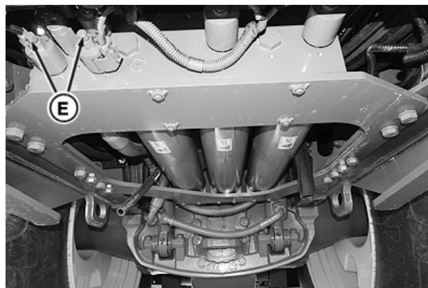
RXA0160220—UN—17JUL17 Electroválvulas hidráulicas (ubicadas debajo del bastidor delantero)
