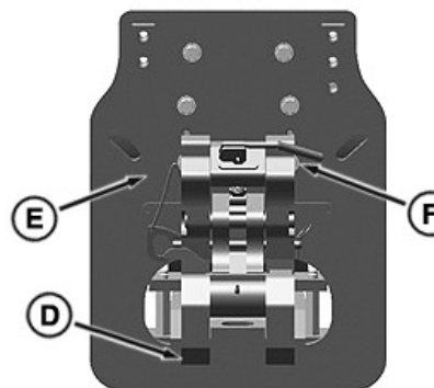
Brzospojna ljljajuća poteznica
