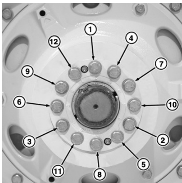
RXA0090157—UN—08AUG06 Redoslijed zatezanja: Sastavljanje zašiljene glavčine pogonskih kotača za oteţane uvjete rada
