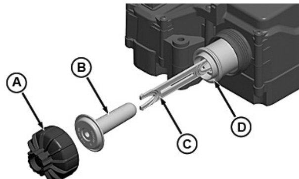
Filter DEF jedinice za doziranje
