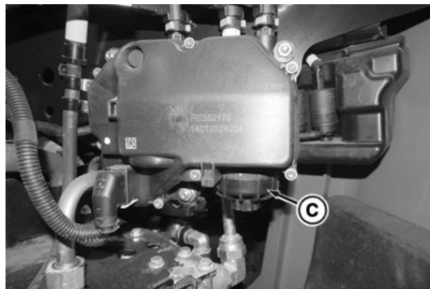
Filter jedinice za doziranje DEF (C) nalazi se u odjeljku akumulatora, pri dnu jedinice za doziranje DEF.
