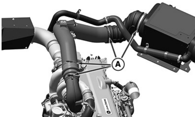
Dubbelturbomotor
