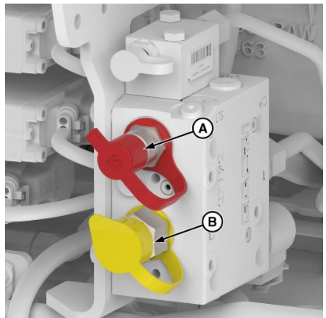
Hydrauliska vagnsbromskopplingar
