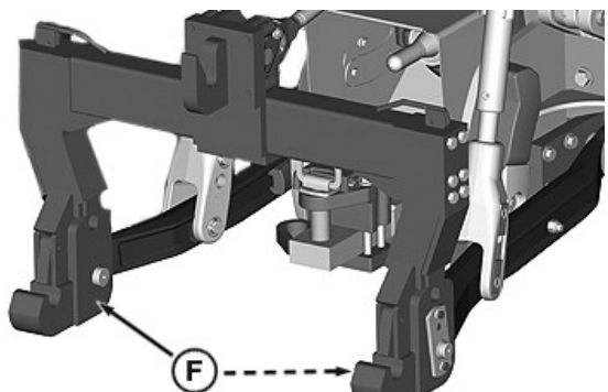
RXA0184147—UN—22JUN21 4N kategorijas konfigurācijā parādīta ātrā sakabe
