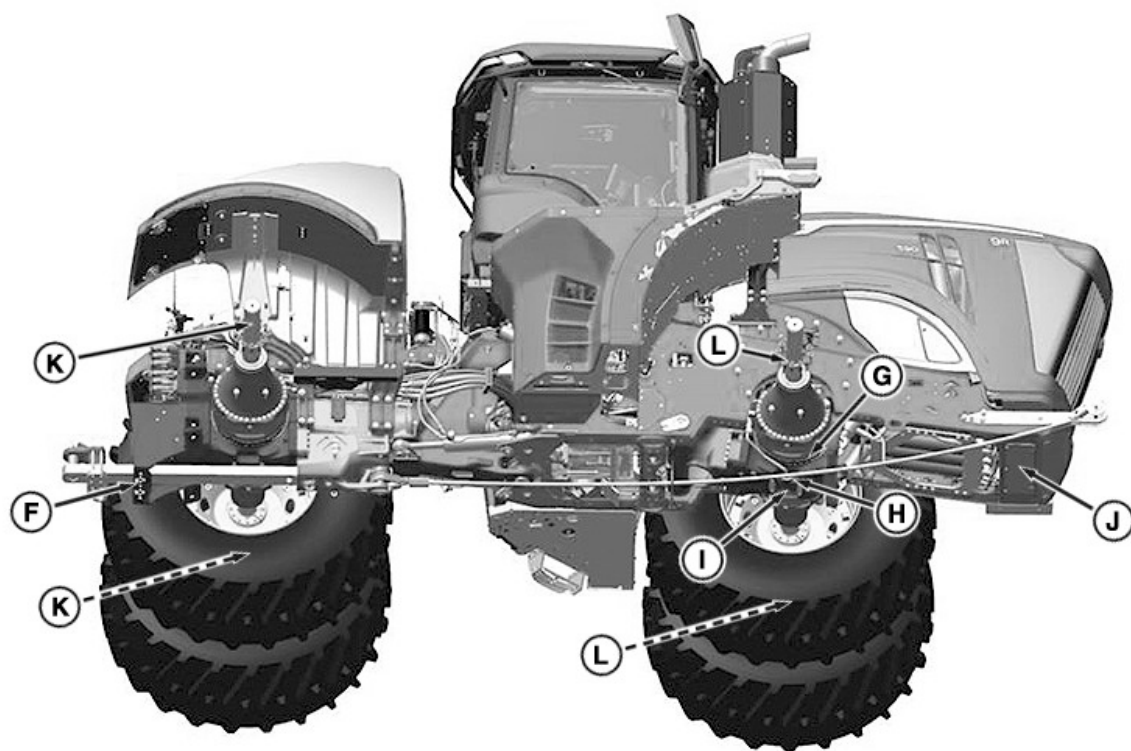
Celšanas punkti (apakšpuse ar [Ag] jūgstieni)
