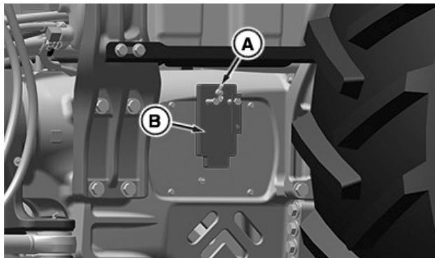
RXA0188394—UN—20DEC22 Stūres iekārtas fiksators uzglabāšanas pozīcijā (kreisā pusē)
