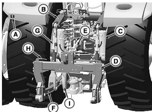
Aizmugurējās sakabes sastāvdaļas
