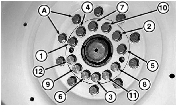
Pievilkšanas secība: Dubultais koniskās lielas noslodzes dubulto riteņu rumbas mezgls
