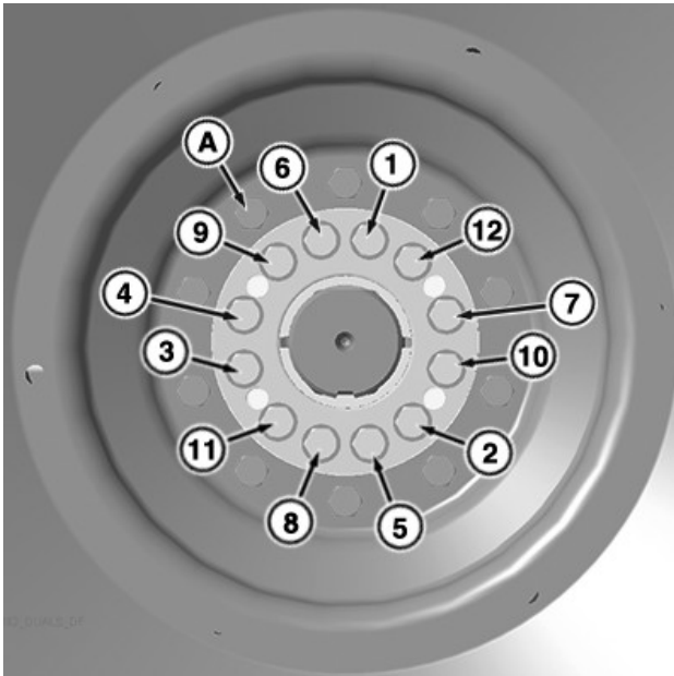
Pievilkšanas secība: Dubultais plakanas lielas noslodzes dubulto riteņu rumbas mezgls
