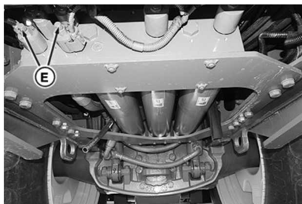
Hidraulikas solenoīdu vārsti (atrodas zem priekšējā rāmja)
