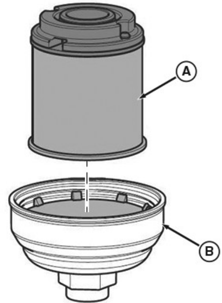
Instalación de la carcasa del filtro y los componentes
