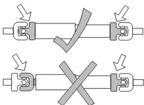
Articulación del eje de transmisión
