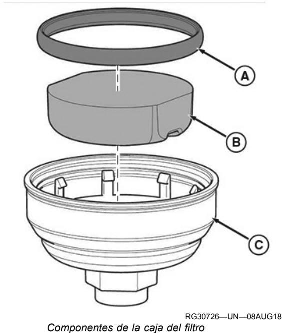
Componentes de la caja del filtro
