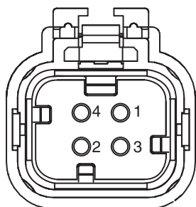
Identification des bornes du connecteur vidéo
