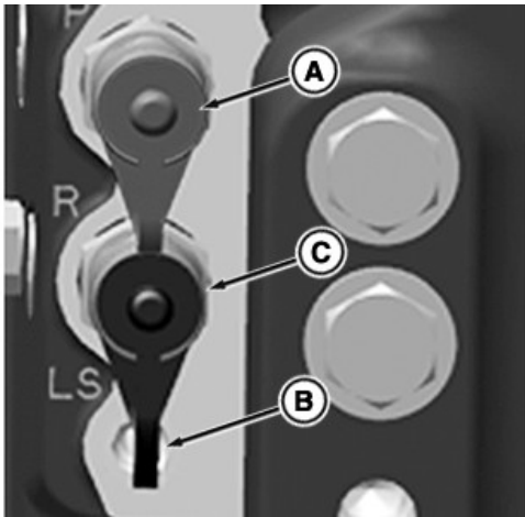
Raccord Power-Beyond—Pièce moulée d'attelage
