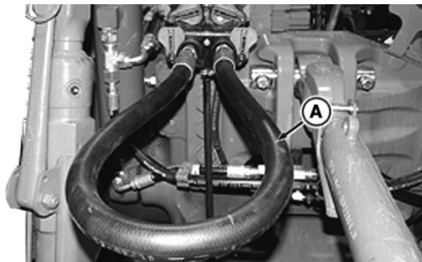
Pose du flexible de raccordement sur le raccord de distributeur auxiliaire [Ag]
