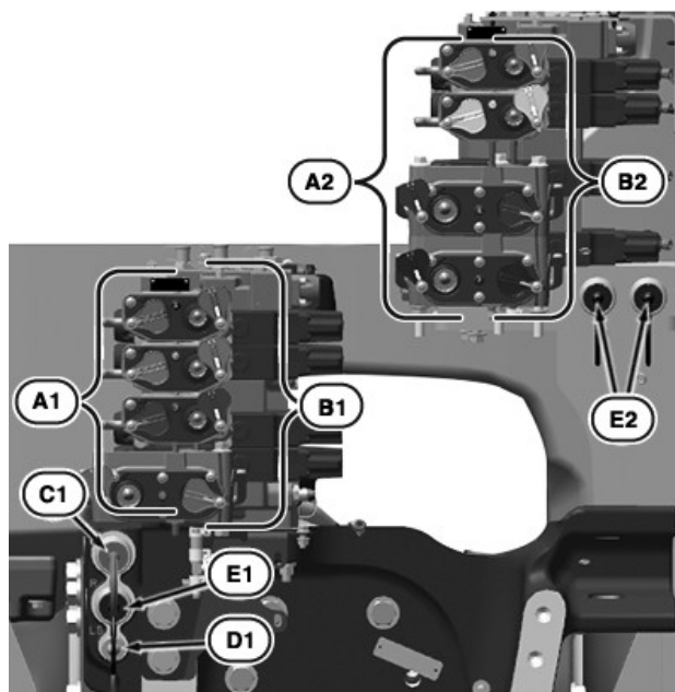
Bloc de distributeurs auxiliaires hydrauliques à haut débit— Huit distributeurs auxiliaires avec Power-Beyond au niveau de la pièce moulée d'attelage
