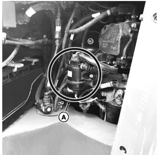
El filtro en línea de fluido de escape diésel (DEF) (A) está dentro del compartimento de la batería.
