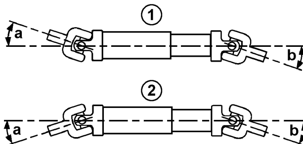
LX1049749—UN—21MAY10 Articulación del eje de transmisión
