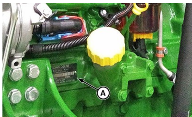
RX1415090—UN—22JUL25 Placa del número de serie del motor (A) (se han retirado las piezas para mayor claridad)
