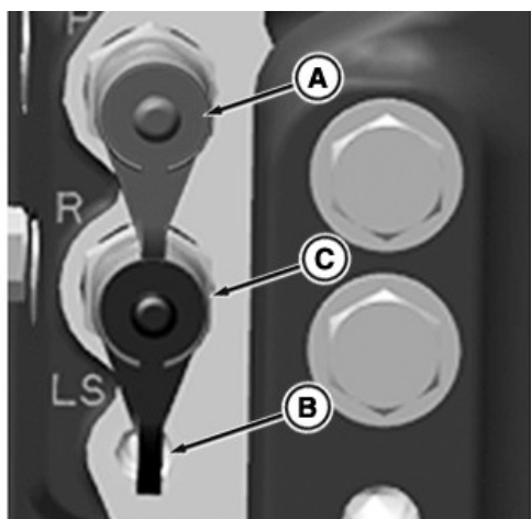
Raccord Power-Beyond—Pièce moulée d'attelage
