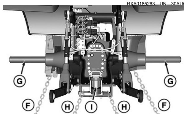
Опора тягово-сцепного устройства и контактная поверхность тягово-сцепного устройства
