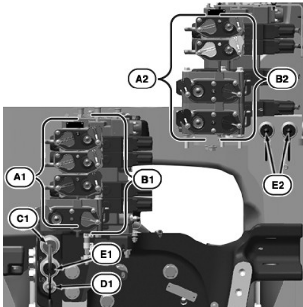
Блок селективных контрольных клапанов гидравлической системы с высоким расходом — восемь селективных контрольных клапанов с Power Beyond в литом компоненте навески
