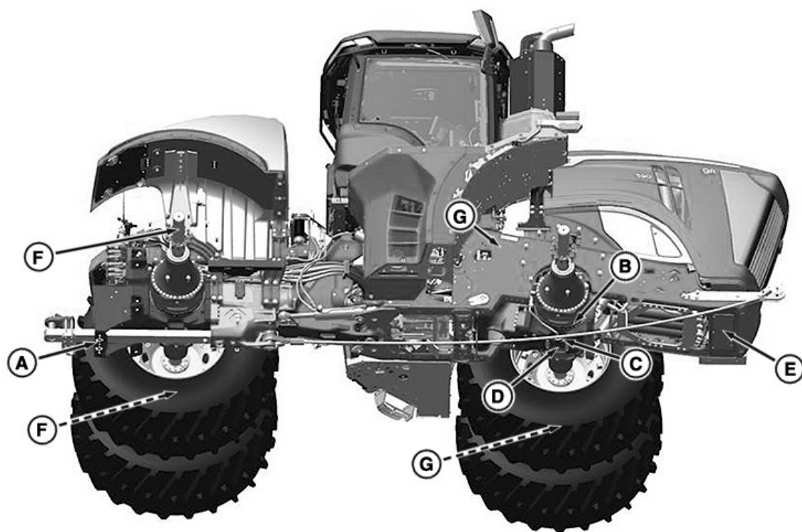
Вид снизу, поддомкратные площадки
