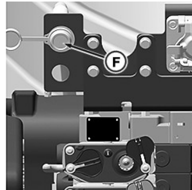
Идентификация компонентов и их расположение [с/х] — гидравлическая система с высоким расходом: (F) Муфта отстойника — слив из корпуса мотора
