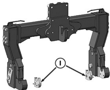
RXA0184178—UN—22JUN21 Attelage rapide avec crochet de catégorie 3 illustré
