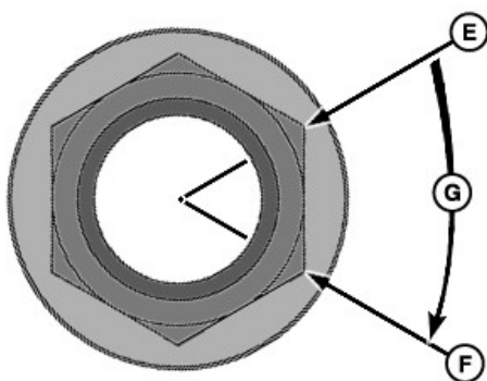
Seção Transversal do Rolo Espigador Exibida
