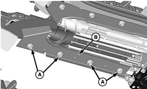
A—Parafuso e Arruela (8 utilizados) B—Lâmina de resíduos (2 usadas)
