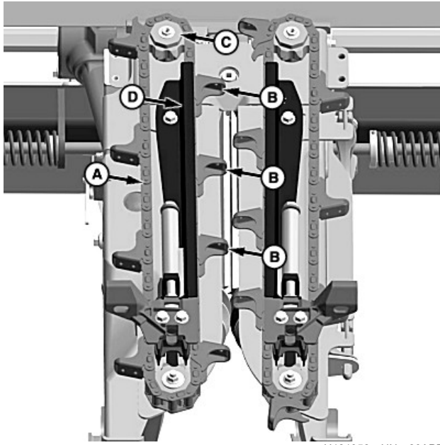
A—Chaîne d'alimentation B—Spires avec l'écartement le plus faible (3) C—Pignon d'entraînement D—Guide de chaîne
