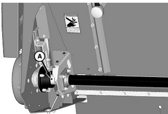
A—Graisseur du limiteur de couple de l'entraînement de la vis d'alimentation
