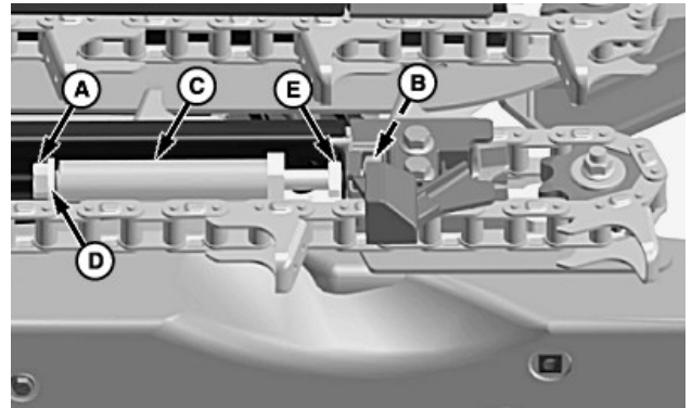
A—Vis B—Écrou C—Tube d'écartement D—Rondelle E—Écrou
