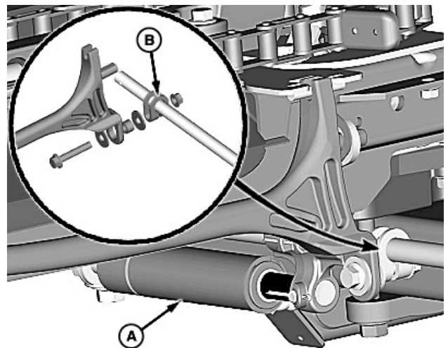
A—Vérin
