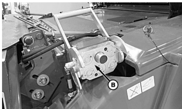
A—Couvercle B—Surface du multicoupleur
