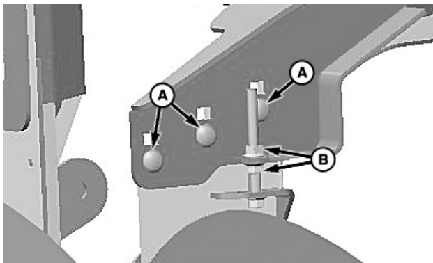
A—Tornillo de carruaje y tuerca (se usan 3) B—Tuerca (se usan 2)
