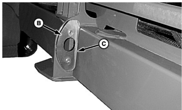
A—Pasador de retención B—Placa de bloqueo C—Bastidor D—Separación inferior E—Separación superior F—Tornillos
