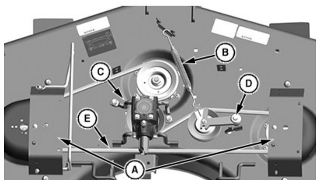
60D Tondeuse (— MY19) illustré, MY20 — similaire
