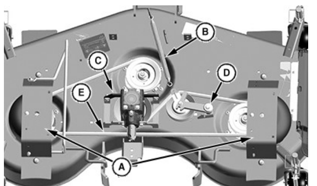
54D Tondeuse (— MY19) illustré, MY20 — similaire
