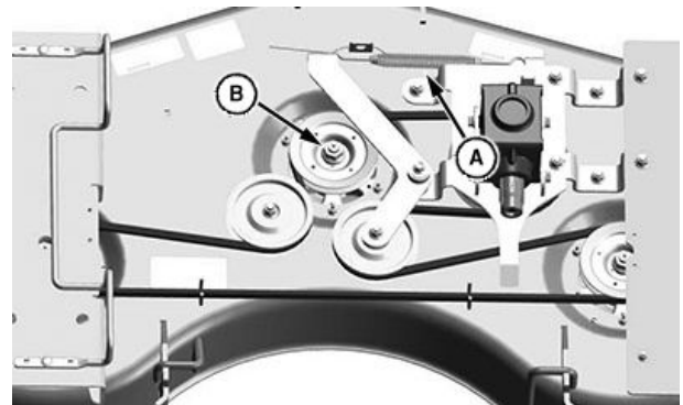
Cortador 60D
