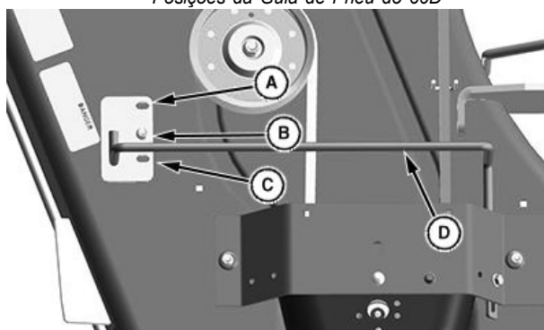
Posições da Guia de Pneu do 72D
