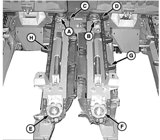
A—Ruedas dentadas traseras B—Ruedas dentadas traseras C—Unidad de hilera D—Unidad de hilera
