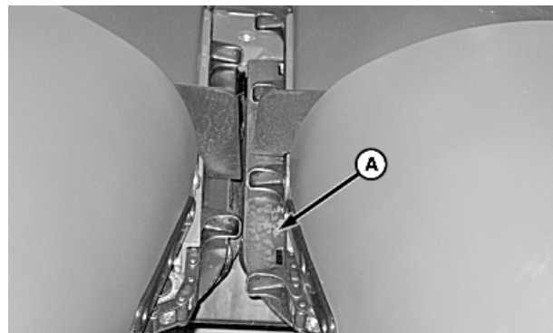
A—Placa de cubierta
