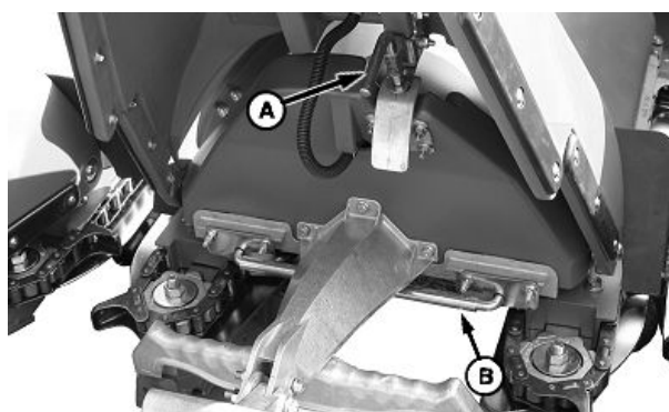
B—Tyč závoru
