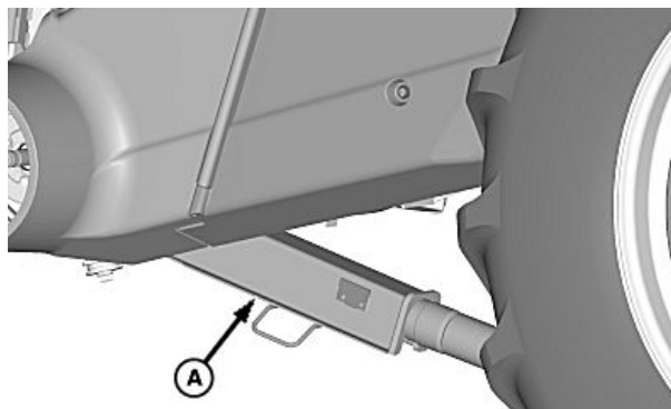
A—Bezpečnostná zarážka
