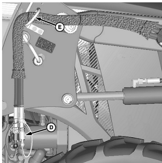
A—Raccord mâle B—Raccord femelle C—Bouchon (4 ou 6) D—Capuchon (4 ou 6) E—Support de flexible
