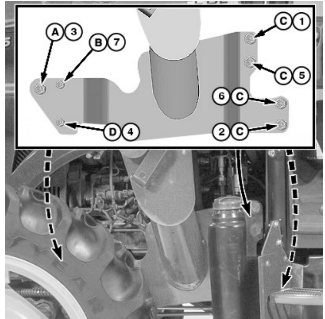
Ordre de serrage (côté gauche illustré)
