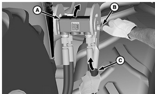
Multicoupleur
