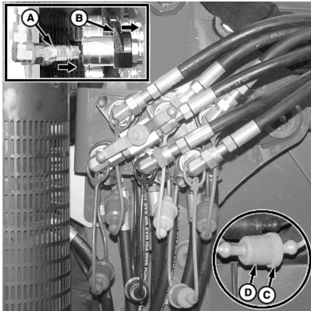
Raccords latéraux
