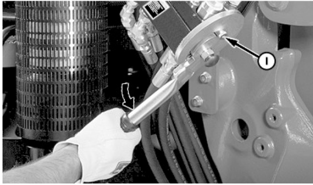
I—Axe (1 de chaque côté)
