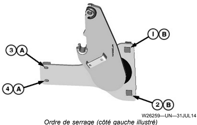
Ordre de serrage (côté gauche illustré)
