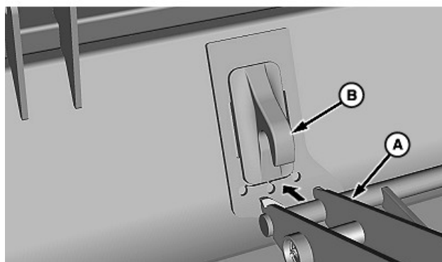
A—Tablier porte-équipement (1 de chaque côté) B—Crochet (1 de chaque côté)
