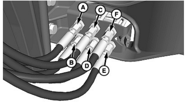
Flexibles au niveau du support de distributeurs latéraux (tracteurs série 5M FT4)
