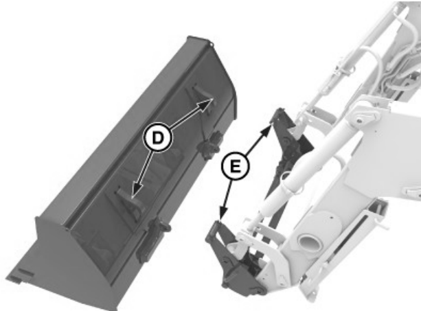
D—Crochet (1 par côté) E—Support (1 de chaque côté)
