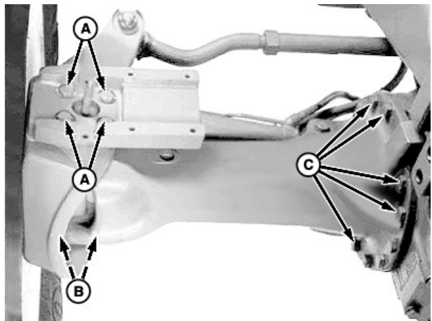
Carter d'essieu côté droit (vu de l'avant)
