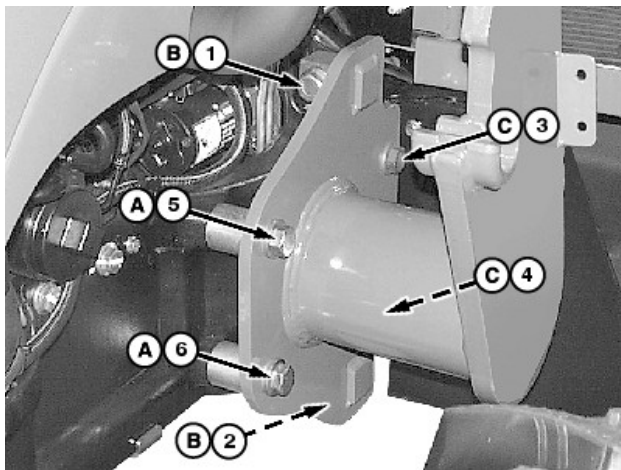
Ordre de serrage (côté gauche illustré)
