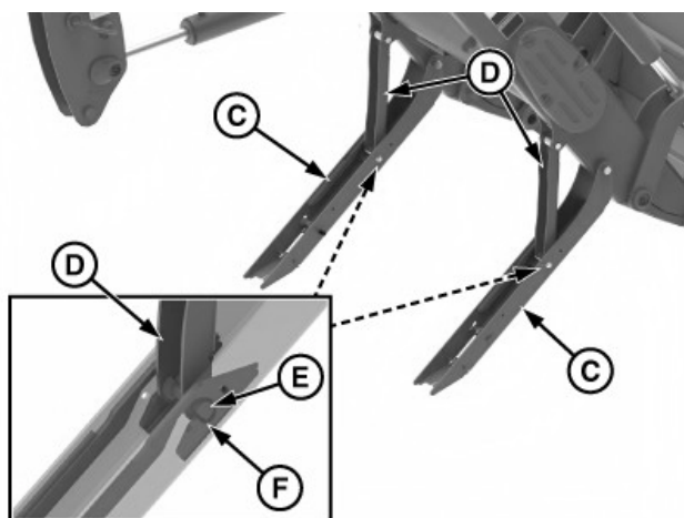
C—Béquille de stationnement (1 par côté) D—Support (1 par côté) E—Axe (1 par côté) F—Crochet (2 par béquille)
