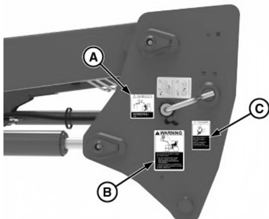
APY88262—UN—08DEC23 Côté gauche (520M sans mise à niveau automatique illustré)
