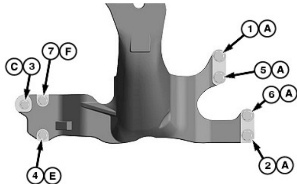
W28948—UN—28SEP20 Ordre de serrage—Côté gauche
