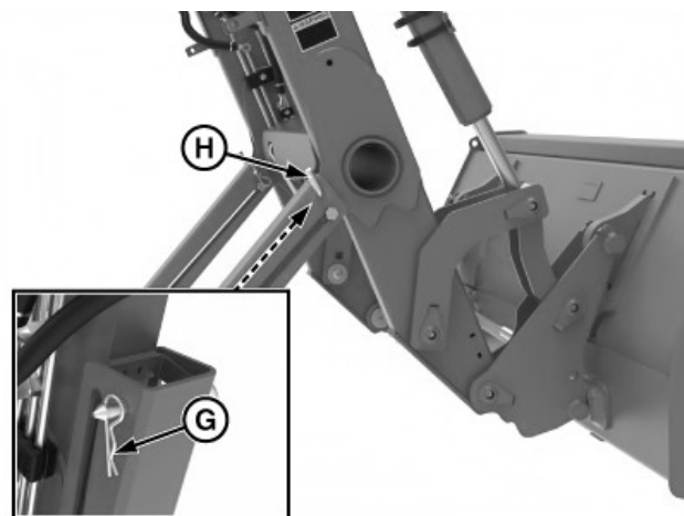
Béquille de stationnement 500M illustrée
