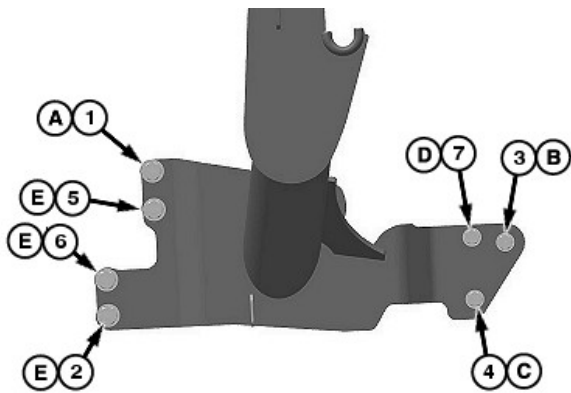
W28137—UN—06JUL17 Ordre de serrage (côté droit)
