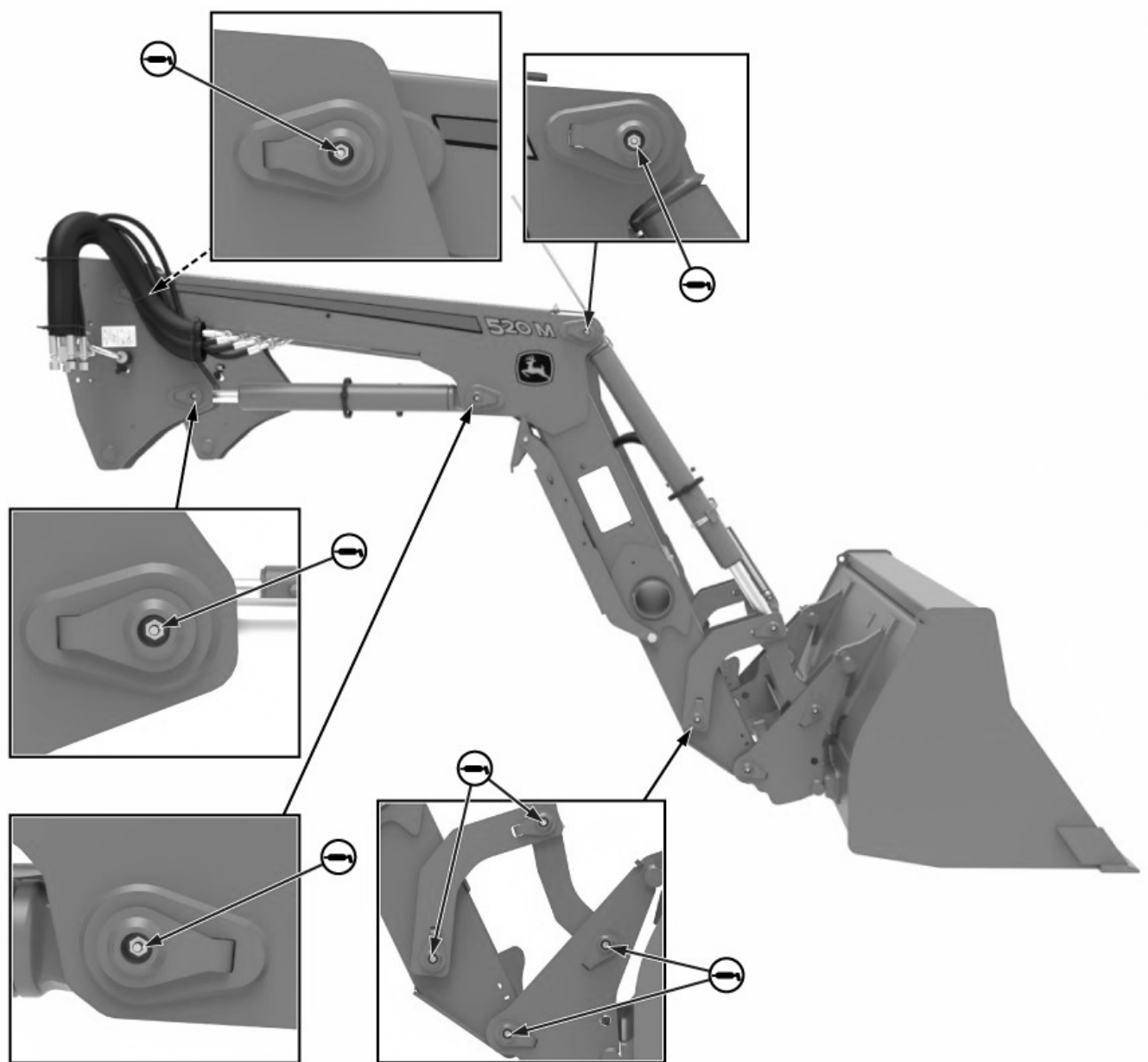
Points de lubrification (520M sans mise à niveau automatique)
