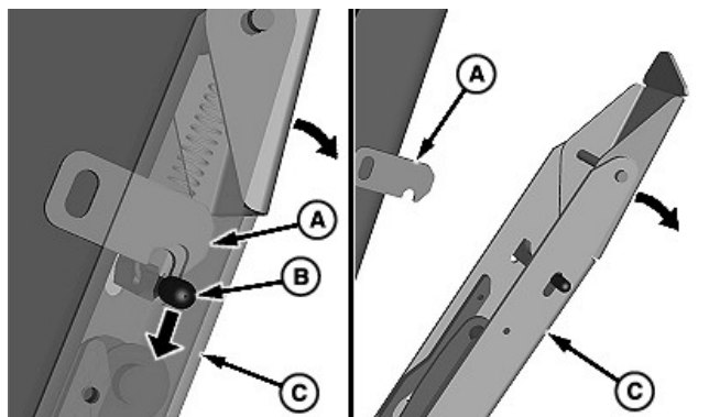
A—Plaque de verrouillage (1 de chaque côté) B—Verrouillage (1 par côté) C—Béquille de stationnement (1 par côté)
