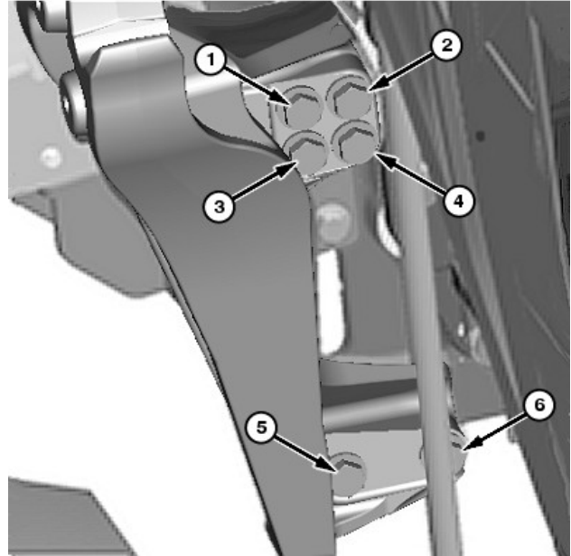
Tracteurs séries 6E et 6D (i4; MA13 et plus récents) (côté droit illustré)
