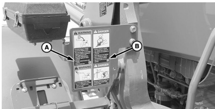
Support de boîte à outils en option—Côté gauche (tracteurs série 5M uniquement)
