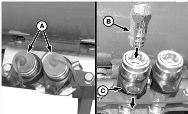
A—Bouchon (2) B—Raccord, mâle C—Raccord, femelle
