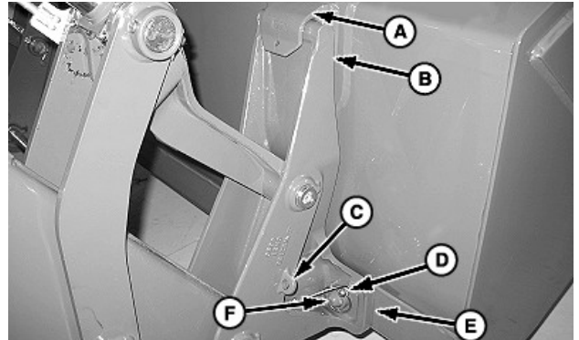
A—Crochet (1 par côté) B—Engin porteur C—Position de rangement D—Goupille à anneau (1 de chaque côté) E—Patte du tablier porte-équipements (1 de chaque côté) F—Axe de benne (1 de chaque côté)
