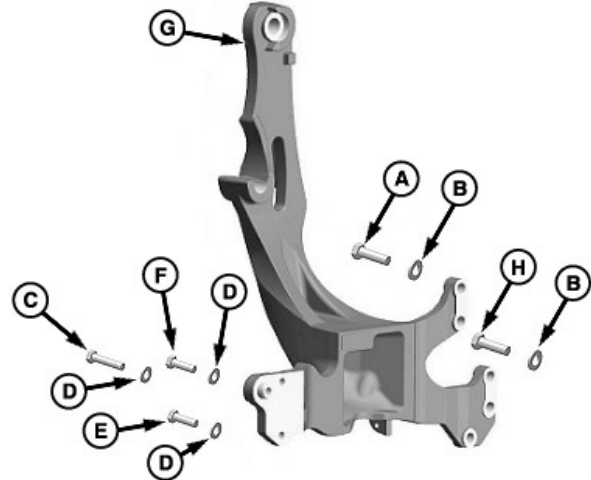
W28947—UN—28SEP20 Côté droit représenté
