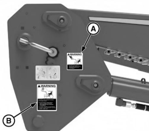
APY88265—UN—08DEC23 Côté droit (500M sans mise à niveau automatique illustré)
