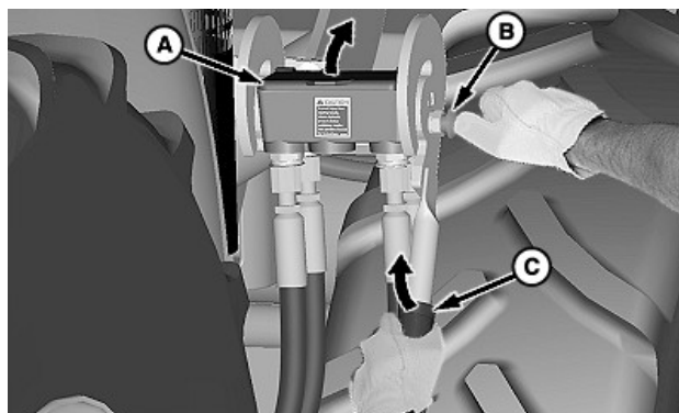
Multicoupleur
