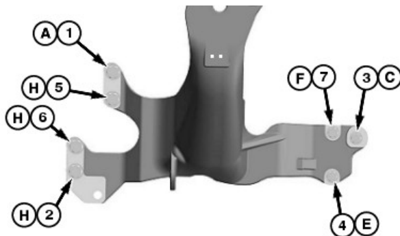
W29371—UN—01JUN22 Ordre de serrage—Côté droit
