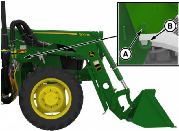
APY88267—UN—23JAN24 500M Loader Shown
