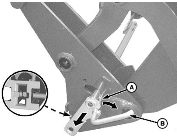
A—Pin B—Handle
