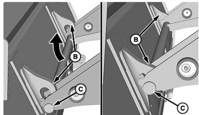
B—Hook (1 per side) C—Bar
