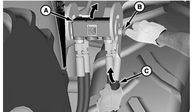
Multicoupler
