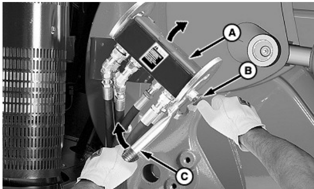
Multicoupler
