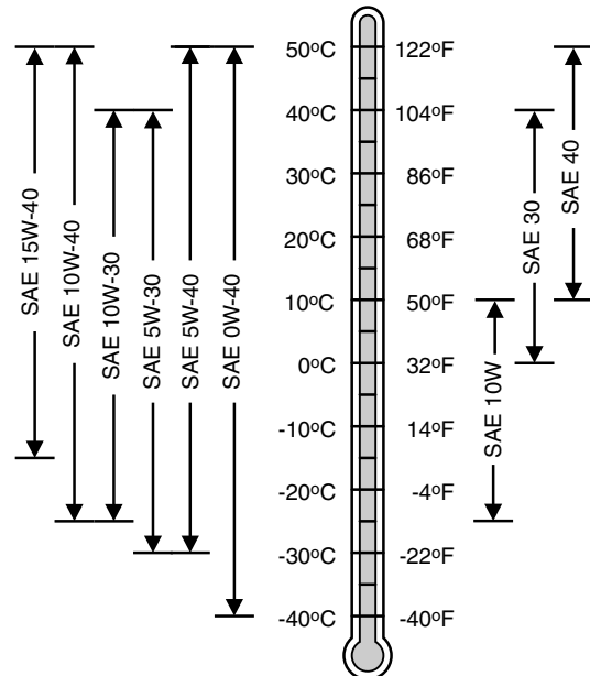
대기 온도 범위에 적합한 오일 점도
