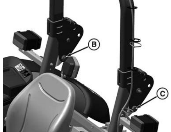
볼트 및 너트 설치
