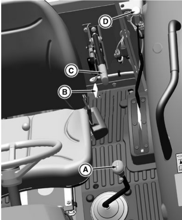
좌측 제어장치
