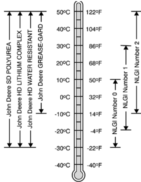
대기 온도 범위에서 사용 가능한 그리스
