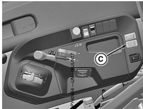
유도등 스위치, 5050E, 5058E, 5067E 및 5075E 만 해당
