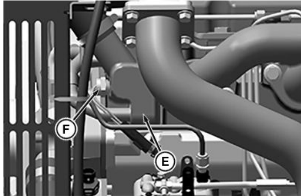
냉각 시동 보조장치 스위치
