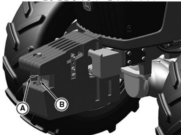
수트케이스 무게추 장착 표준 무게추 지지대
