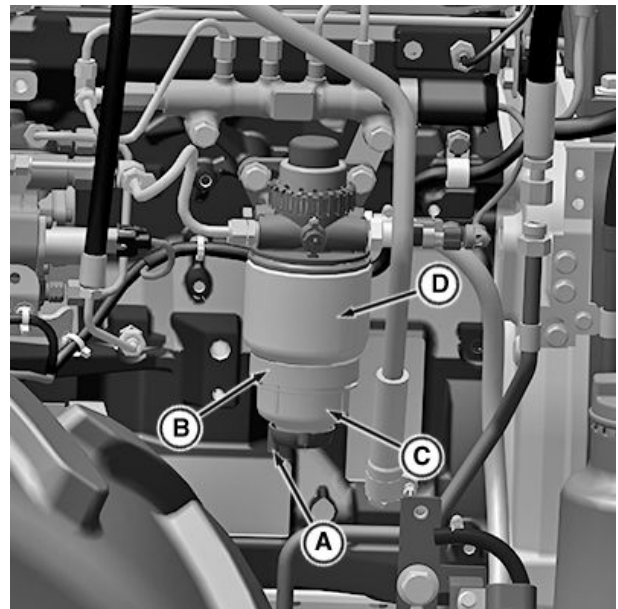
A—드레인 포트 B—하단 고정 링
