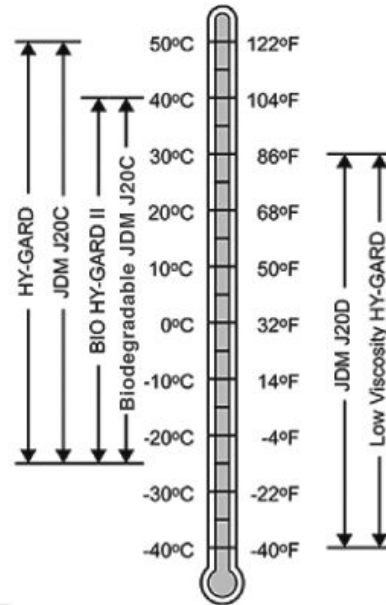
기온 범위별 사용 오일
