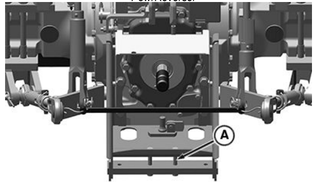
SyncShuttle™
