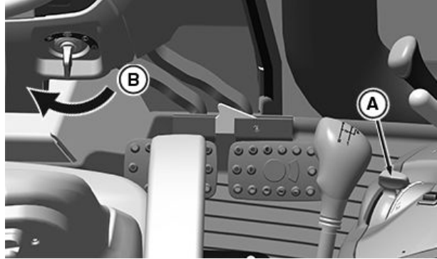
운전실 캡 및 IOOS(캡 장착 가능 개방형 작업자 스테이션) 트랙터, 5050E, 5058E, 5067E 및 5075E
