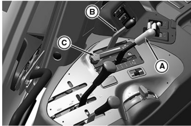
제어 레버, 5050E, 5058E, 5067E 및 5075E 운전실 캡
