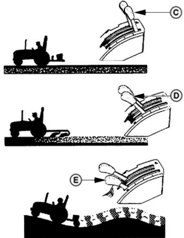
특샤프트 위치 제어
