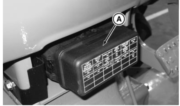
IOOS(캡 장착 가능 개방형 작업자 스테이션), 퓨즈 박스 위치
