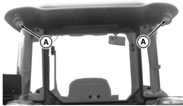
후방 작업등
