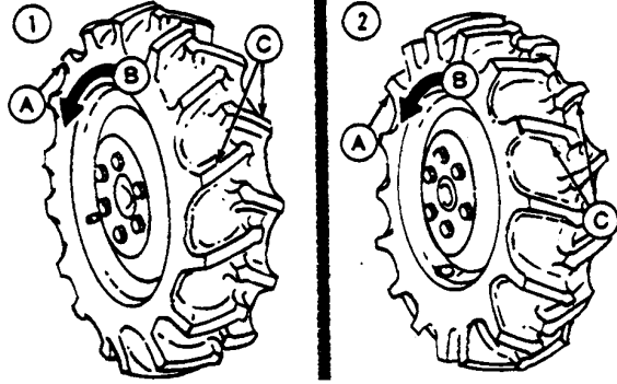
좌측 타이어(뒤에서 본 모습)
