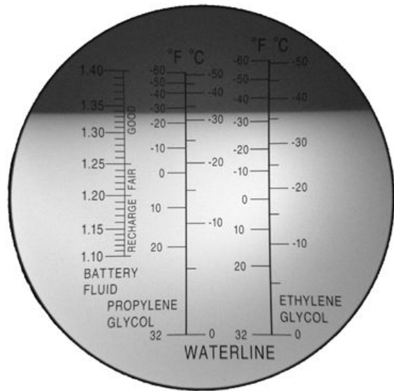
굴절계 창 위에 떨어뜨린 50/50 냉각수 한 방울의 이미지
