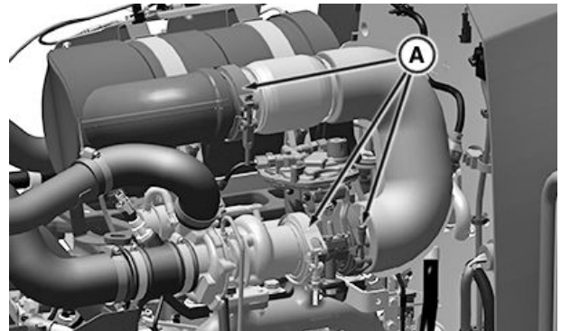
터보차저에서 DOC/DPF
