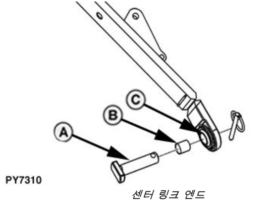
A—마스트 핀 B—센터 링크 부싱
