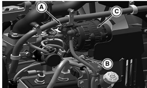
교류 발전기/팬 벨트 조정, 5050E, 5058E, 5067E 및 5075E 운전실 캡 및 IOOS(캡 장착 가능 개방형 작업자 스테이션)만 해당
