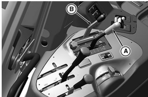
제어 레버, 5058E, 5067E 및 5075E 운전실
