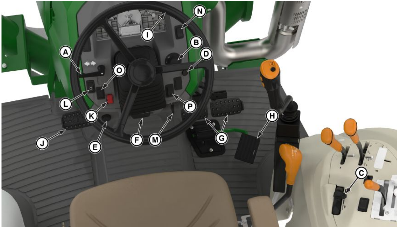
트랙터 제어장치
