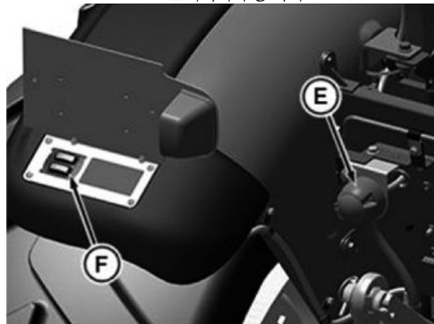
트랙터의 후방 좌측
