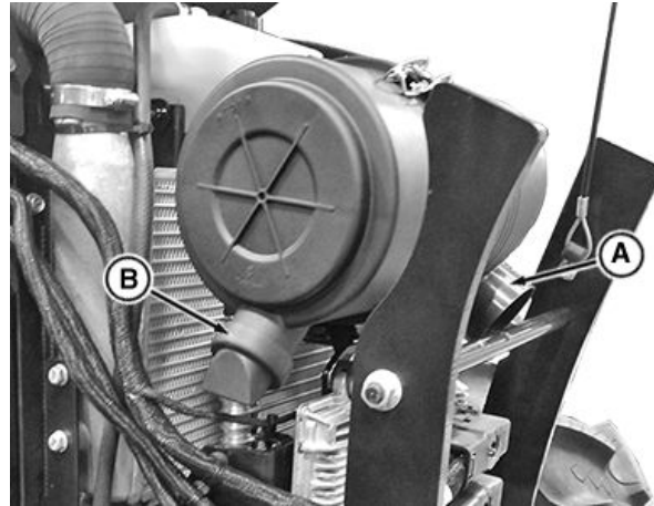
에어 클리너
