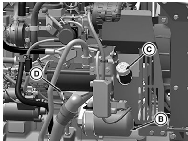
오일 필터, 5050E, 5058E, 5067E 및 5075E 만 해당
