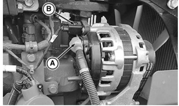
와이어 연결, 5050E, 5058E, 5067E 및 5075E 모델 - IOOS(캡 장착 가능 개방형 작업자 스테이션) 및 운전실 캡
