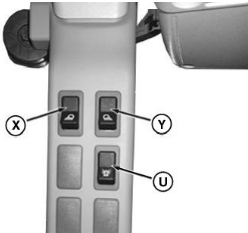
우측 제어장치
