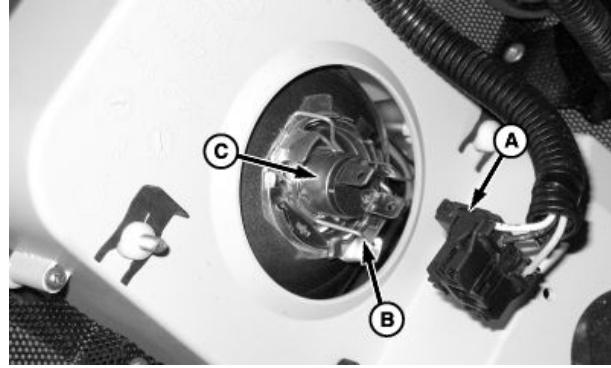
A—커넥터 B—클립
