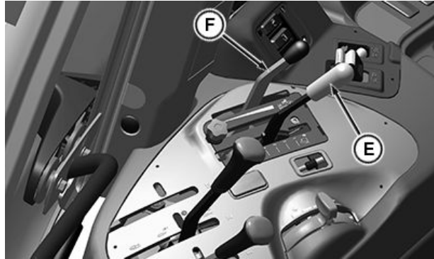
제어 레버, 5058E, 5067E 및 5075E 운전실
