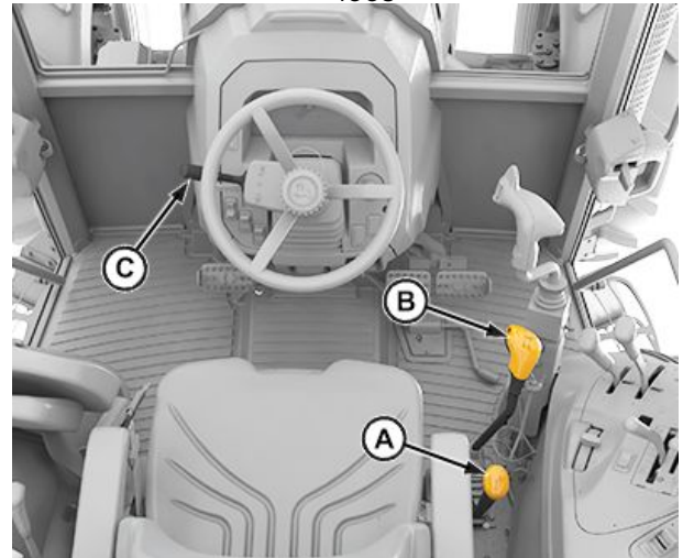
운전실 캡
