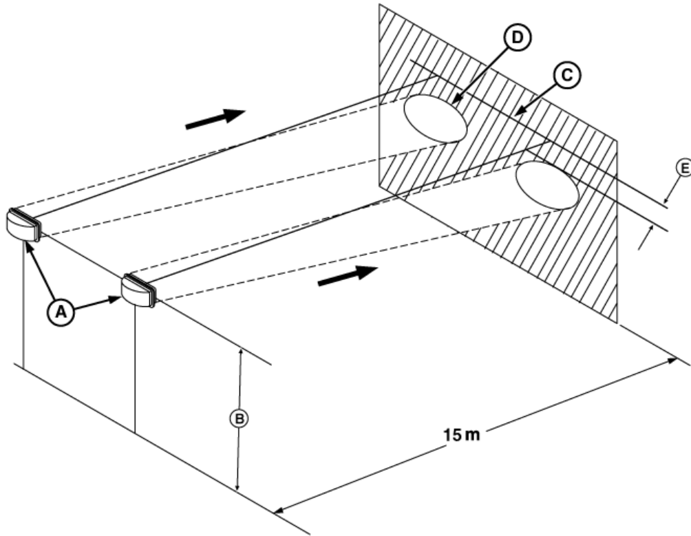
전조등 조준 다이어그램
