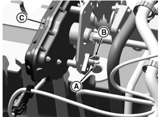
EQRL 조정
