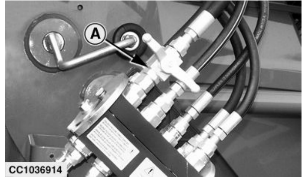
멀티 커플러
