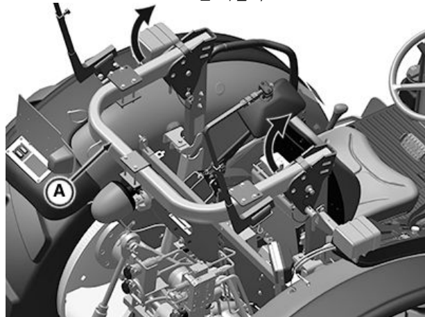
ROPS - 접힘
