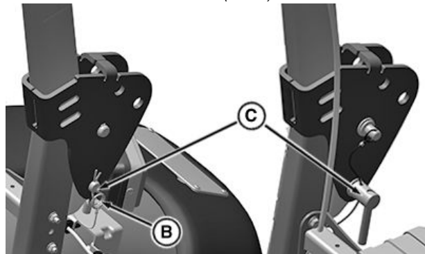
핀 재설치
