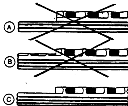
Sección transversal de correa
