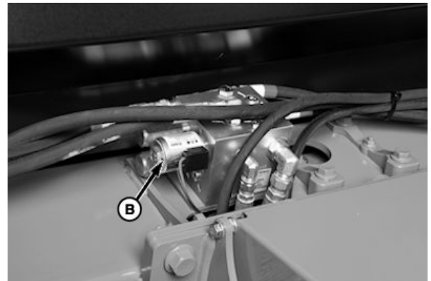
A—Sensor de diámetro de paca B—Electroválvula
