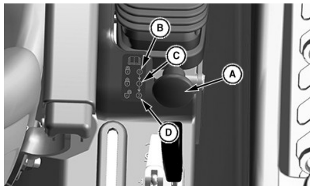
LV28322—UN—11MAY17 A—Verrou du levier de distributeur auxiliaire B—Position 0 C—Position 1 D—Position 2
