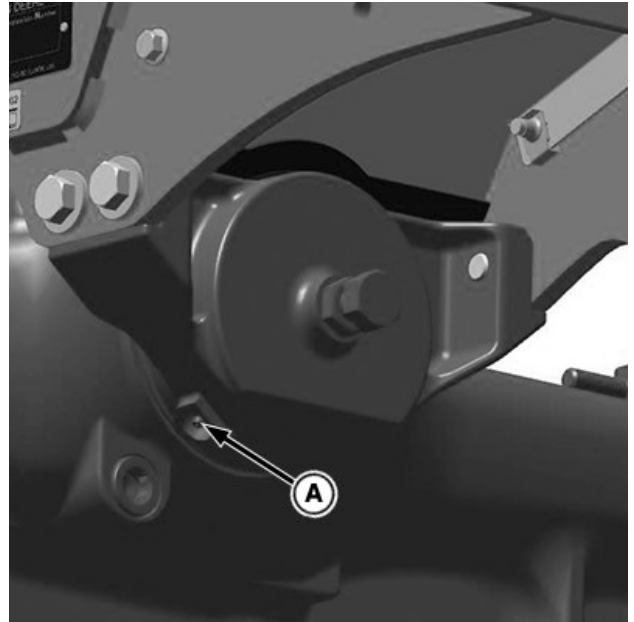
Axe d'attelage à usage intensif
