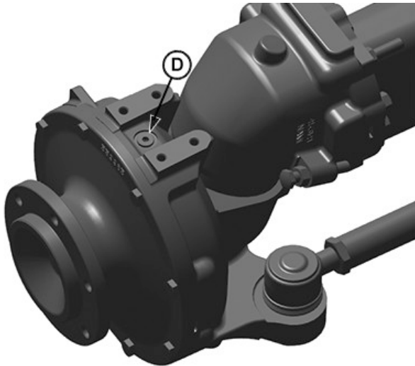
LVP18349—UN—09JAN24 Évent de l'essieu avant renforcé
