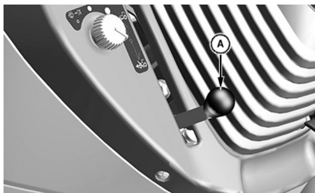
LV29126—UN—09AUG17 Levier du pont avant mécanique de la cabine
