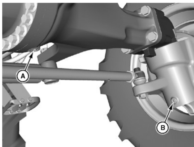
Bouchon de vidange d'essieu avant standard
