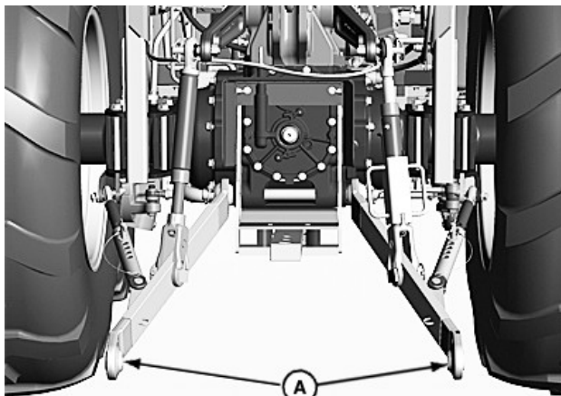
A—Barres de traction
