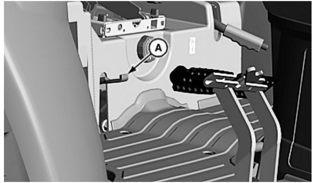
Blocage du différentiel de la boîte PowrReverser
