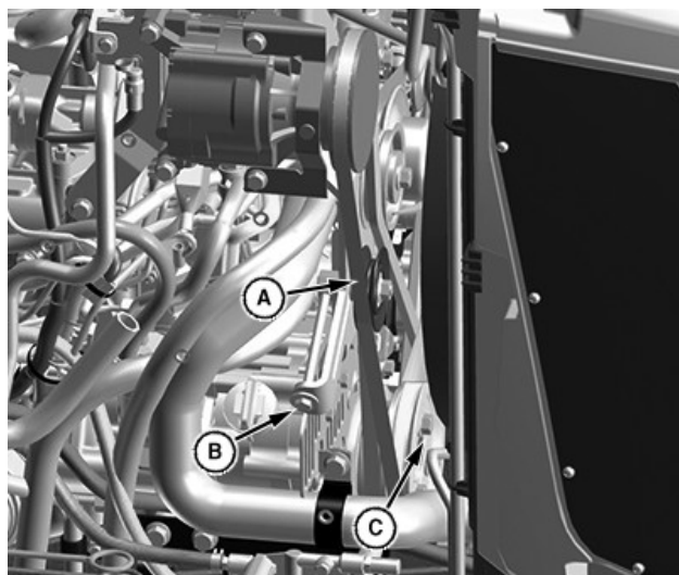
Déposer la courroie
