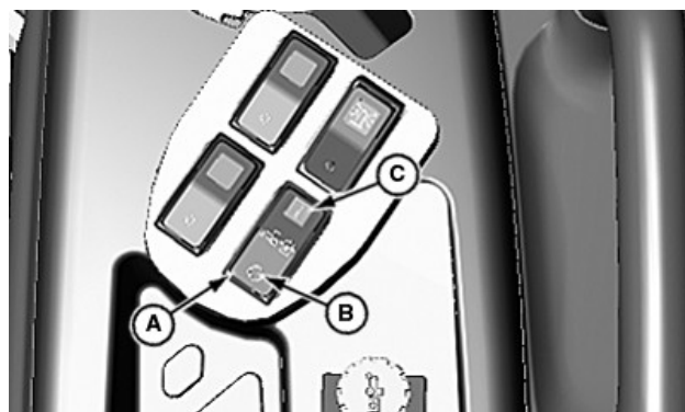
Contacteur de commande de distributeur auxiliaire d'un tracteur de série M illustré (à transmission hydrostatique uniquement)
