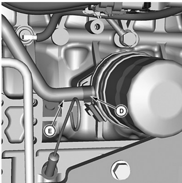
Flexible de liquide de refroidissement moteur, suivant équipement.
