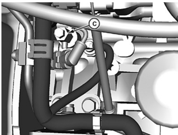
Bouchon de vidange du liquide de refroidissement moteur, suivant équipement.
