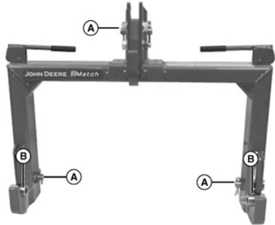
A—Pasador perforado (se usan tres) B—Casquillo (se usan dos)
