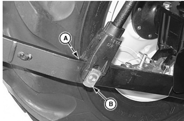
Posición de flotación
