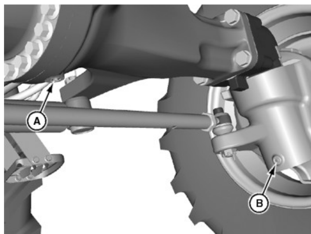
Tapón de vaciado del eje delantero estándar
