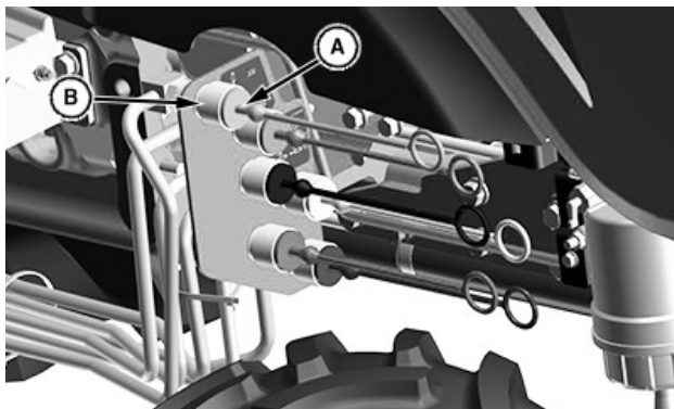
Acopladores de válvula de mando a distancia de posición central
