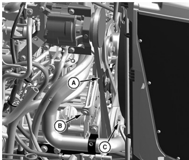
Separación de la correa
