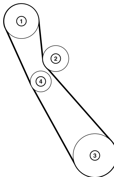
Tendido de la correa
