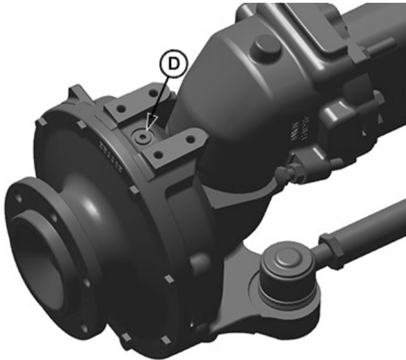
Tapón del respiradero del eje delantero reforzado
