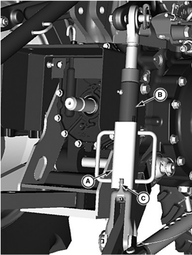
A—Collarín del tensor B—Tensor lateral C—Bloqueo del collarín del tensor
