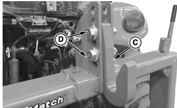
C—Gancho de tensor central D—Tuercas y pernos
