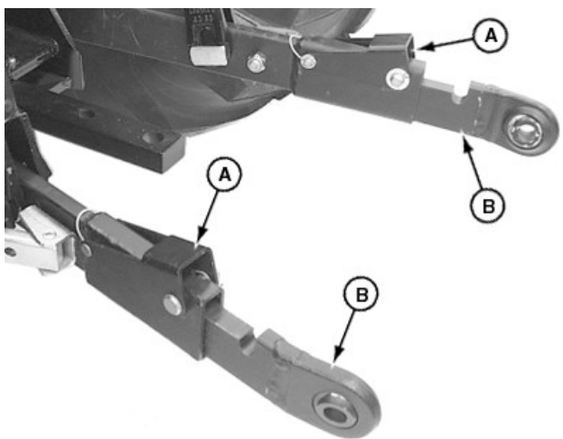
A—Levier de verrouillage B—Lien
