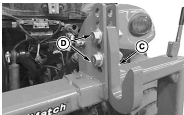
C—Crochet de barre de poussée D—Écrous et boulons
