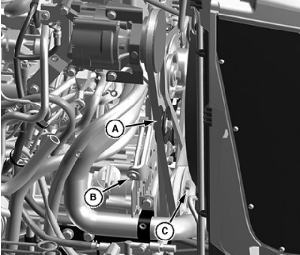
Dépose de la courroie
