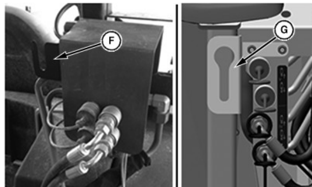
F—Support de rangement pour les tracteurs à cabine ouverte G—Support de rangement pour les tracteurs à cabine
