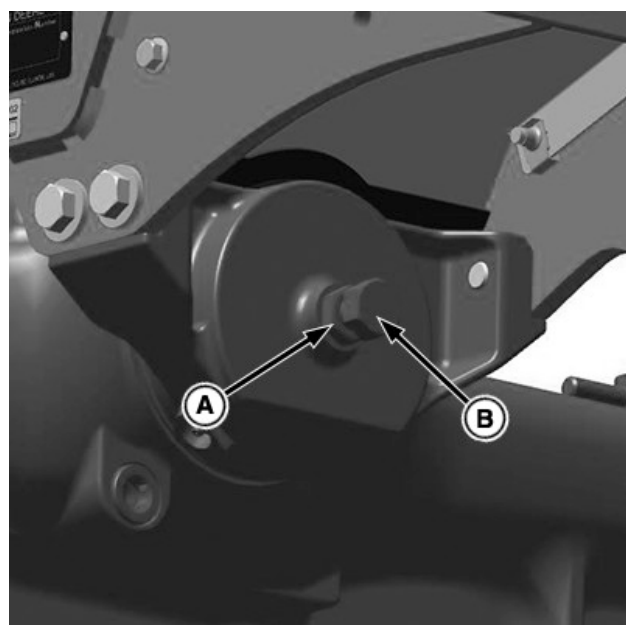
LV30816—UN—03MAY23 Axe d'attelage à usage intensif
