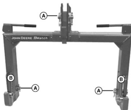
A—Axe percé (3) B—Bague (2)
