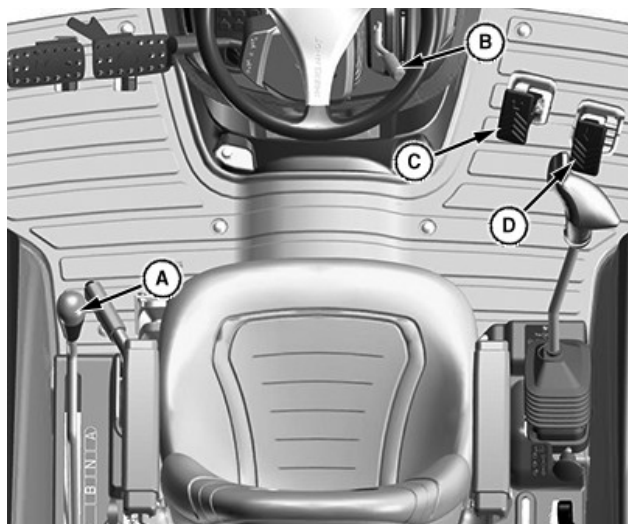
Plate-forme de conduite
