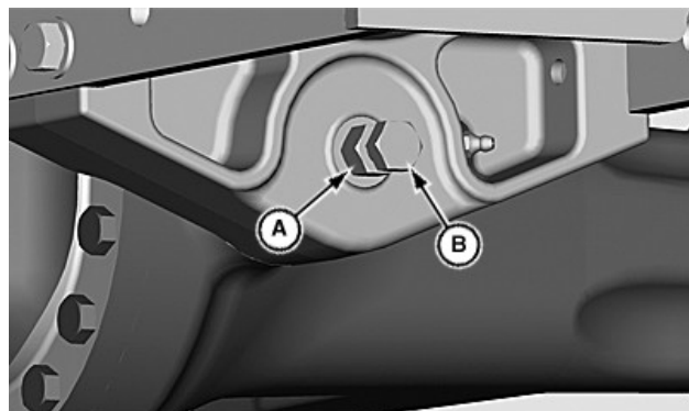
LV19180—UN—26SEP13 Essieu standard
