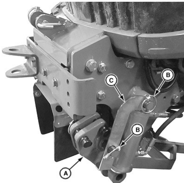
A—Cadre de levage B—Goupilles élastiques C—Supports
