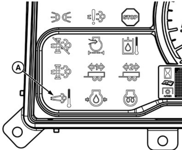
A—Témoin de température élevée du système d'échappement
