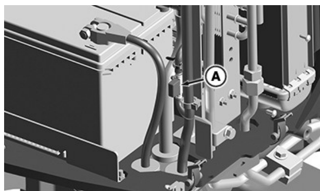
Plate-forme de conduite — Zone de calandre avant près de la batterie — Fusible 30 A
