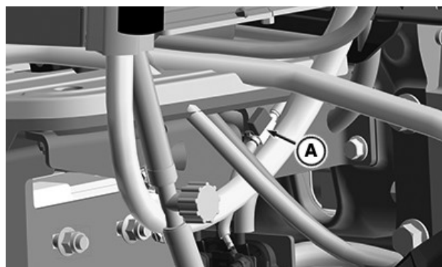
Cabine — Côté droit de la cabine près du compartiment de batterie — Fusible 30 A
