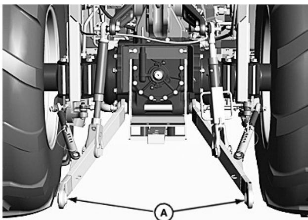
A—Barres de traction
