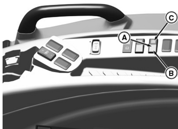
Contacteur de commande de distributeur auxiliaire d'un tracteur de série M illustré (à transmission hydrostatique uniquement)
