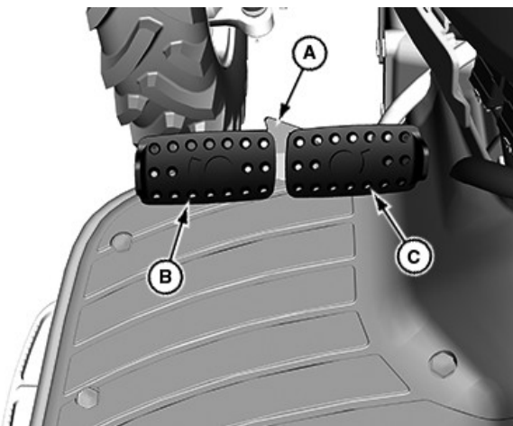
LV17509—UN—19APR13 Pédales de frein de la transmission hydrostatique
