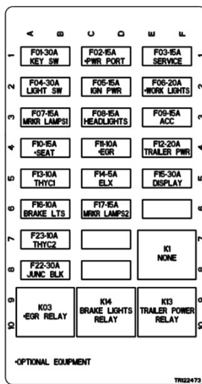
Plataforma de conducción abierta - TR122473
