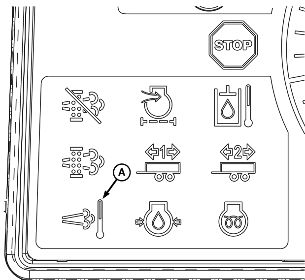
A—Indicador de temperatura de escape alta
