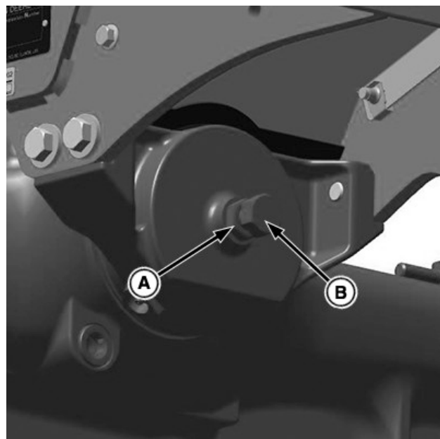
Eje reforzado
