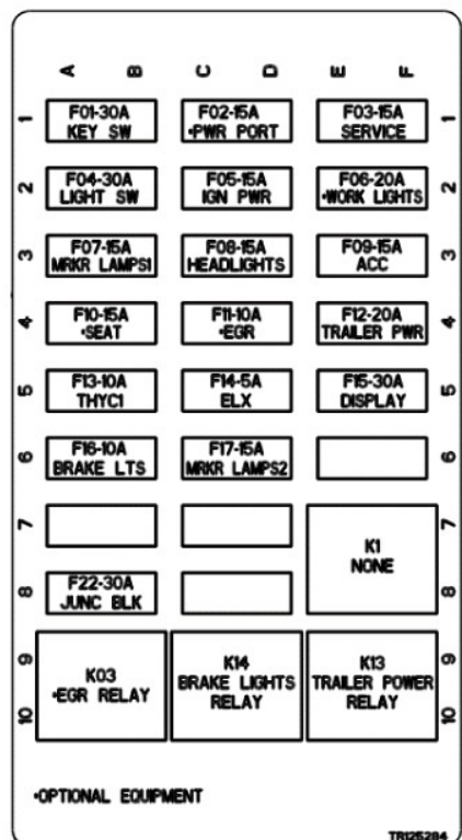
Plataforma de conducción abierta - TR125284
