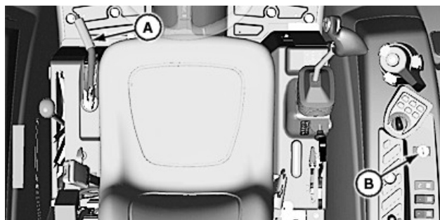
A—Freno de estacionamiento B—Interruptor de la TDF
