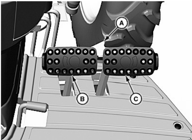
Pedales de freno de la transmisión PowrReverer
