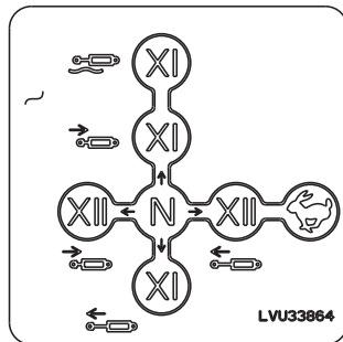
Etiqueta de la válvula de control
