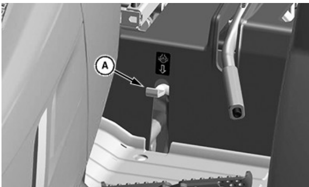
Bloqueo del diferencial de la transmisión hidrostática
