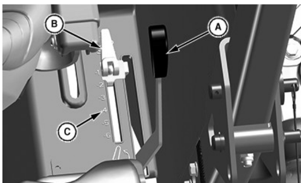
Palanca de control del eje elevador de la plataforma de conducción abierta
