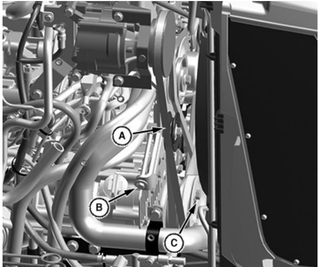
Extracción de la correa
