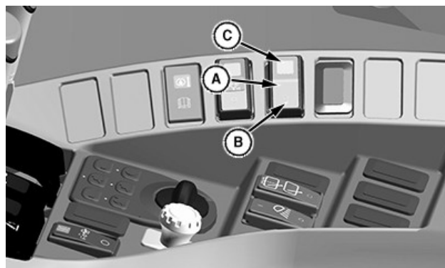
Interruptor de control selectivo—Imagen de la cabina del tractor
