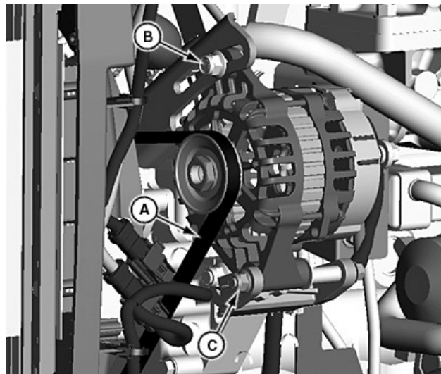
A—Posición del pulgar B—Perno de ajuste C—Perno de pivote
