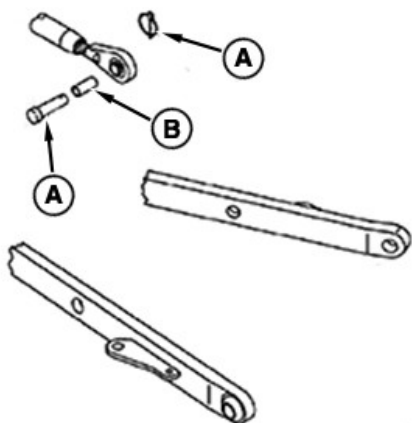
A—Pasador del accesorio B—Casquillo reductor del tensor central
