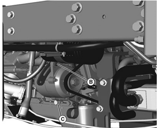
TCAL45057—UN—14MAY13 휘발유 모델 그림. 디젤 모델 엔진 반대편의 교류 발전기입니다. 사진의 선명도를 위해 일부 부품이 제거됨.
