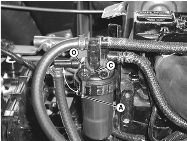
개방 위치의 연료 차단 밸브 그림
