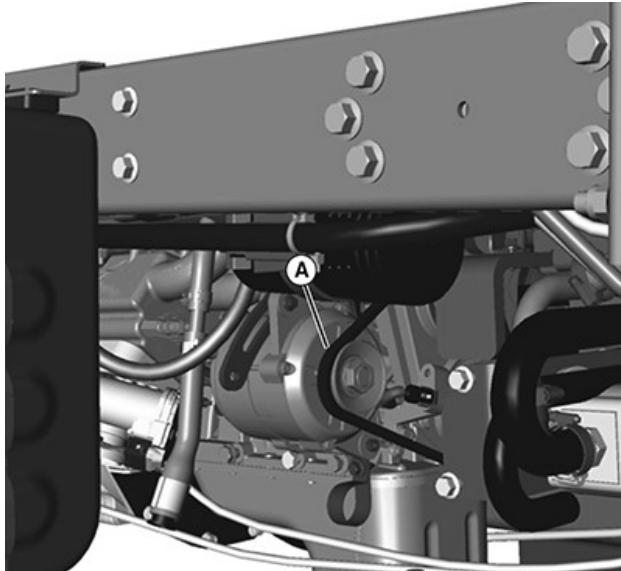
TCAL45056—UN—14MAY13 휘발유 모델 그림. 디젤 모델 엔진 반대편의 교류 발전기입니다. 사진의 선명도를 위해 일부 부품이 제거됨.
