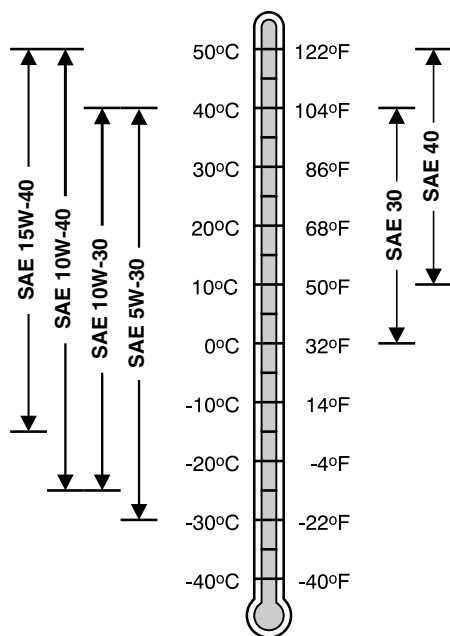
気温範囲に適したオイル粘度
