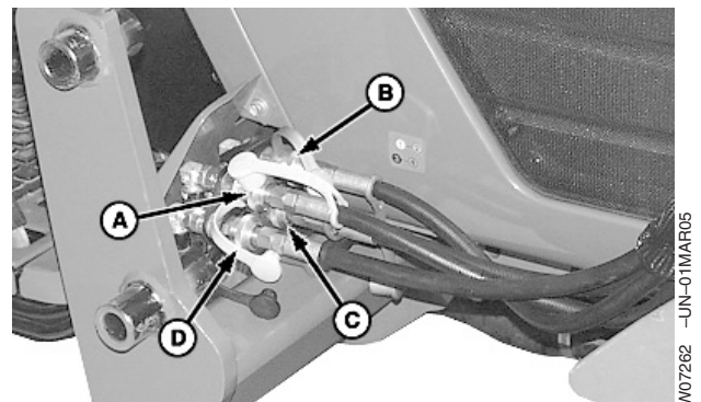
Raccords pour tracteurs 4100, 4110 et 4115
