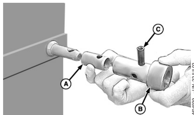
A—Bague B—Bague C—Goupille élastique
