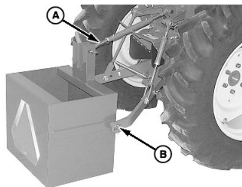
A—Boulonnerie de fixation de la barre de poussée B—Goupille à anneau (2)
