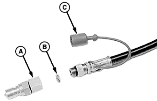
A—Raccord adaptateur B—Restricteur C—Bouchon (VERT ou BLEU)
