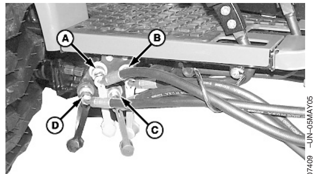
Raccords pour tracteurs 2320, 2520 et 2720
