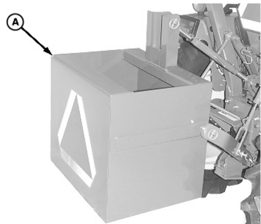
Attelage 3 points avec caisson de lestage
