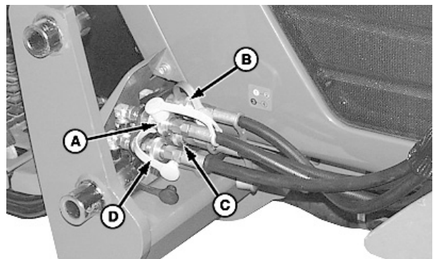
Kupplung der Traktoren 4100, 4110 und 4115
