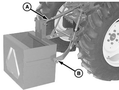
A—Befestigungsteile des Oberlenkers B—Schnappstift (2 St.)
