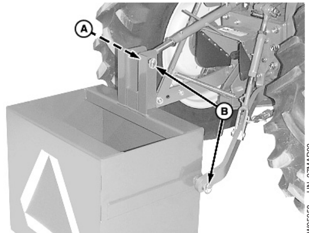
A—Zentrale Verbindung B—Schnappstifte (3 St.)
