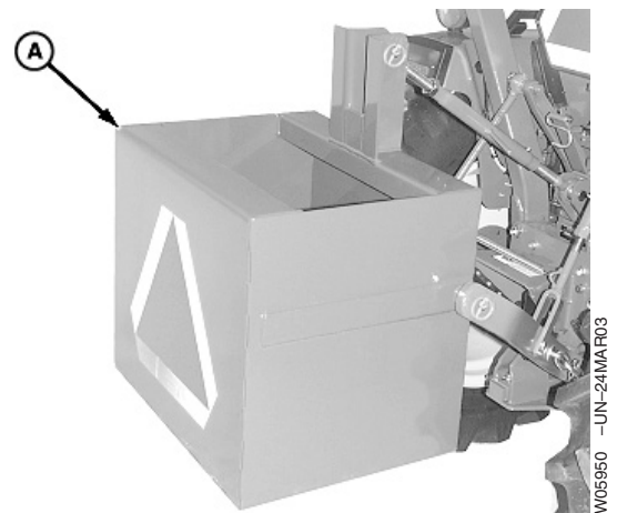
A—Zusatzgewichtkasten
