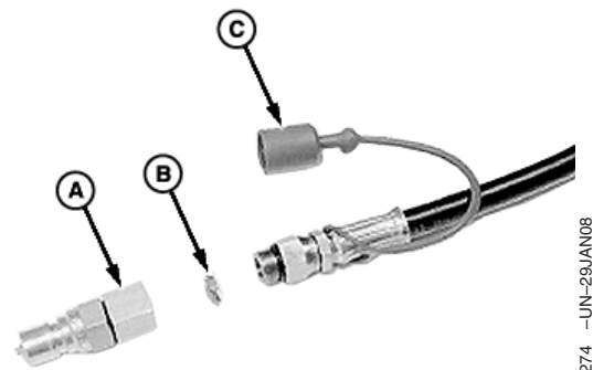
A—Verbindungsanschluß B—Drosselscheibe C—Kappe (GRÜN oder BLAU)
