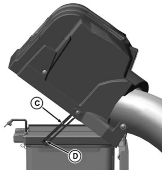
Ανοικτή κατάσταση πάνω μέρους χοάνης
