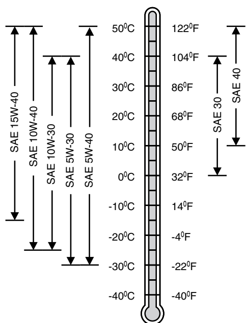
不同气温范围内机油的粘度
